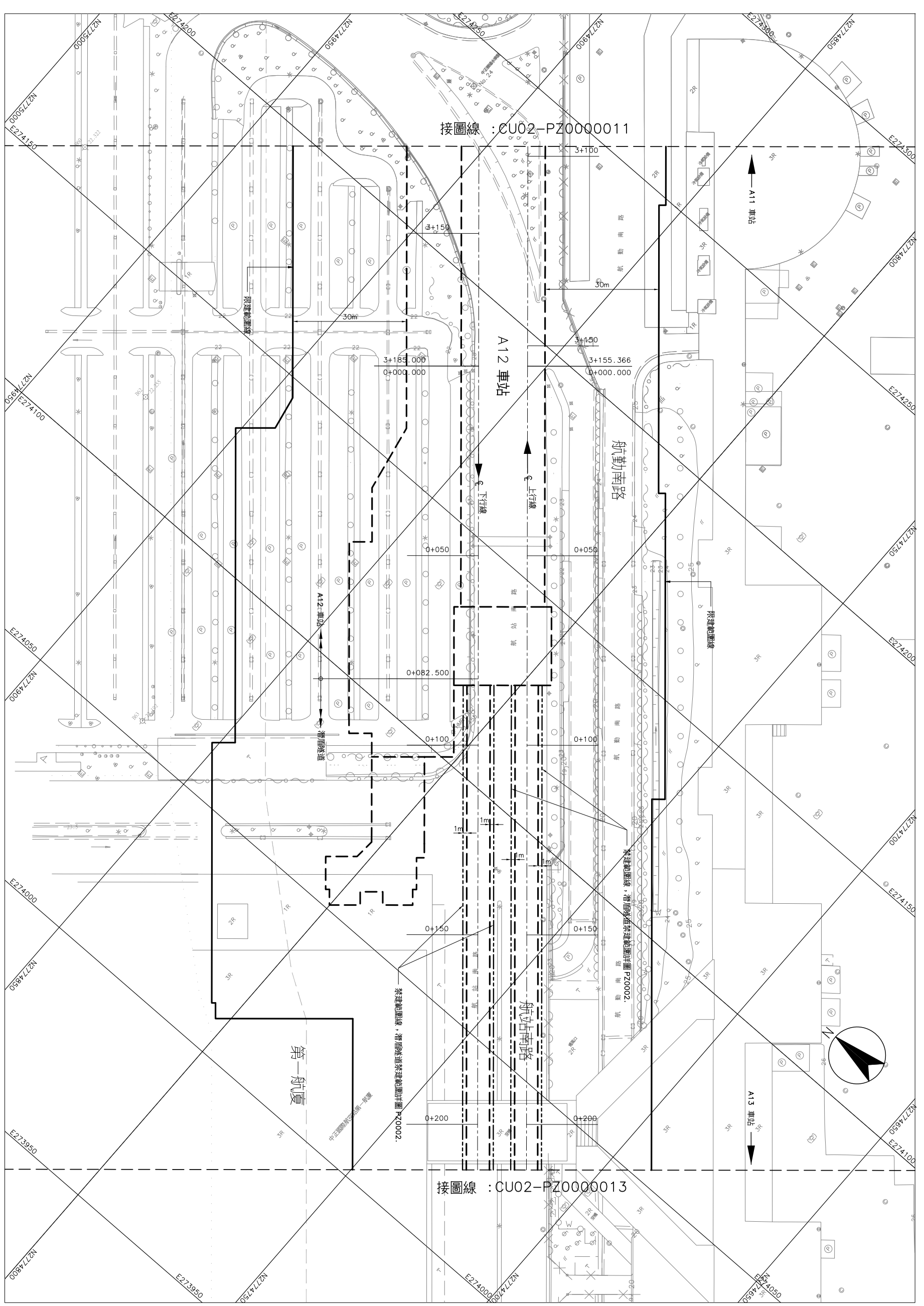
平面圖
