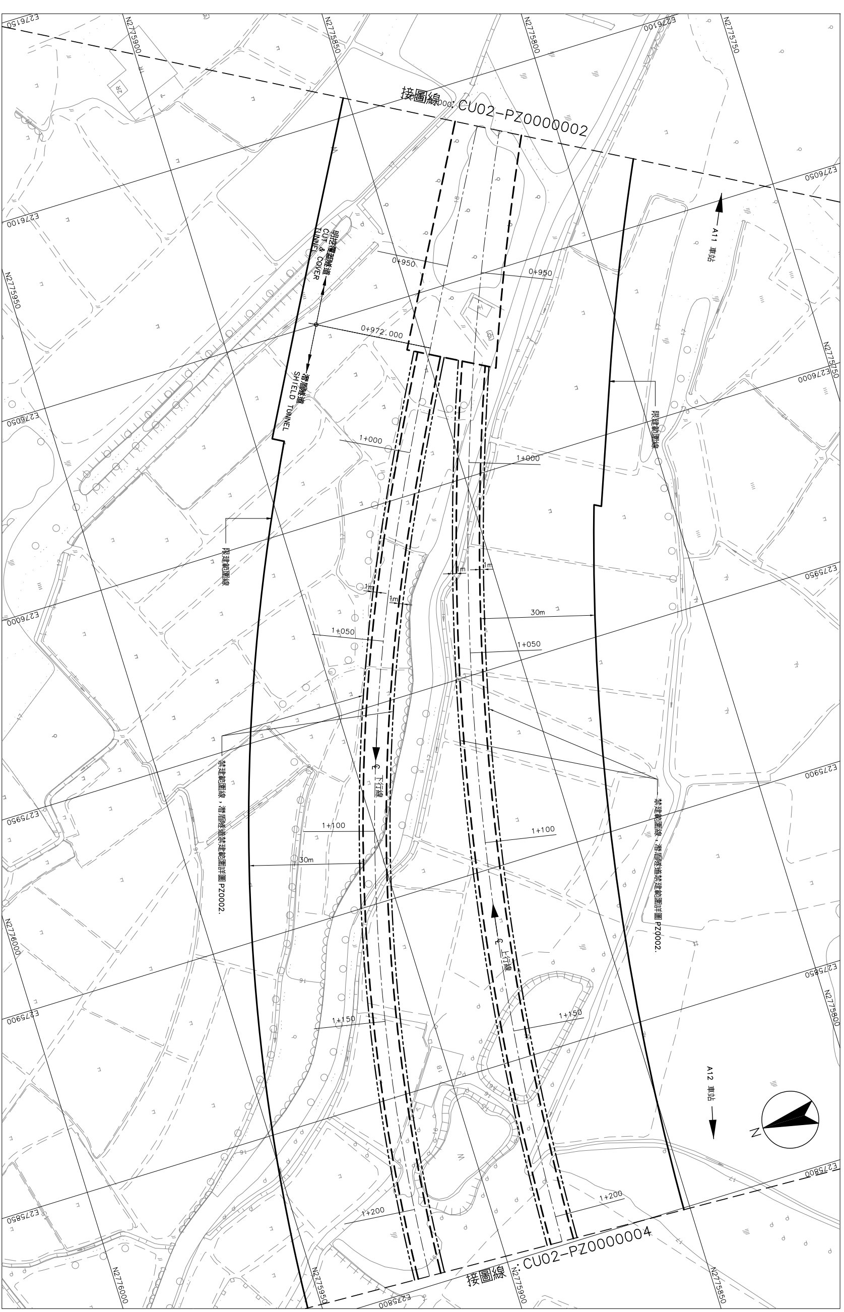
平面圖
