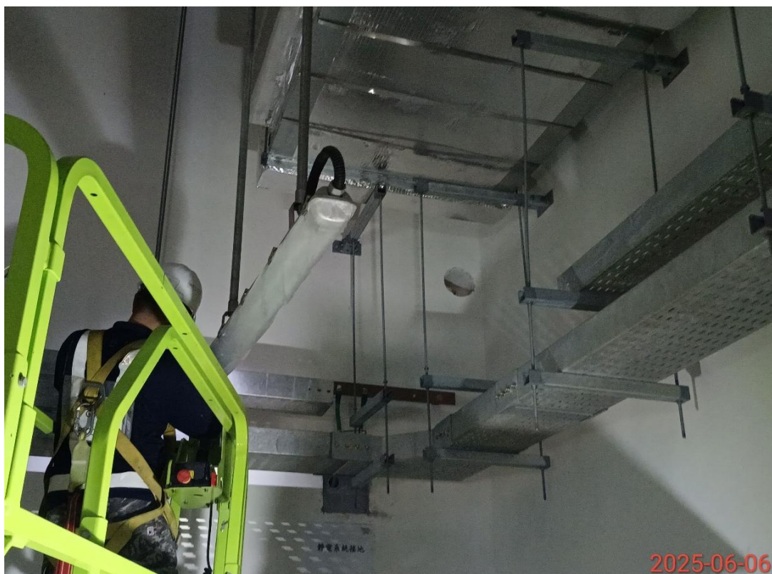
G15 站通訊系統管槽施作
