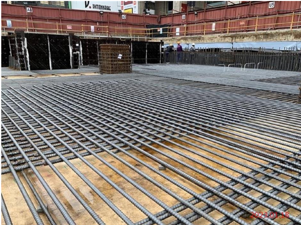
G07 站_站體結構 1FL 柱牆鋼筋綁紮
