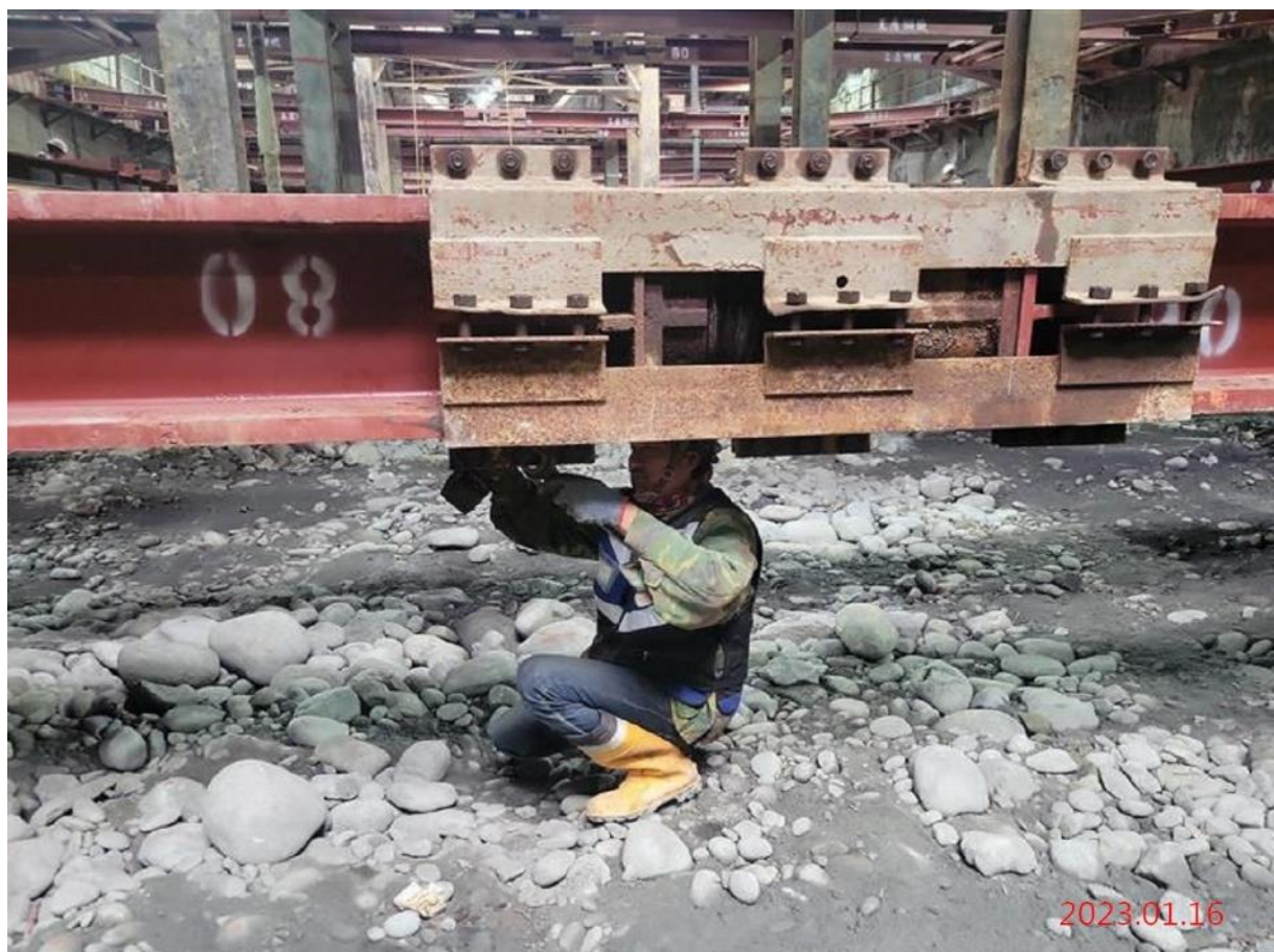
G10 站_南工區第三層支撐施作
