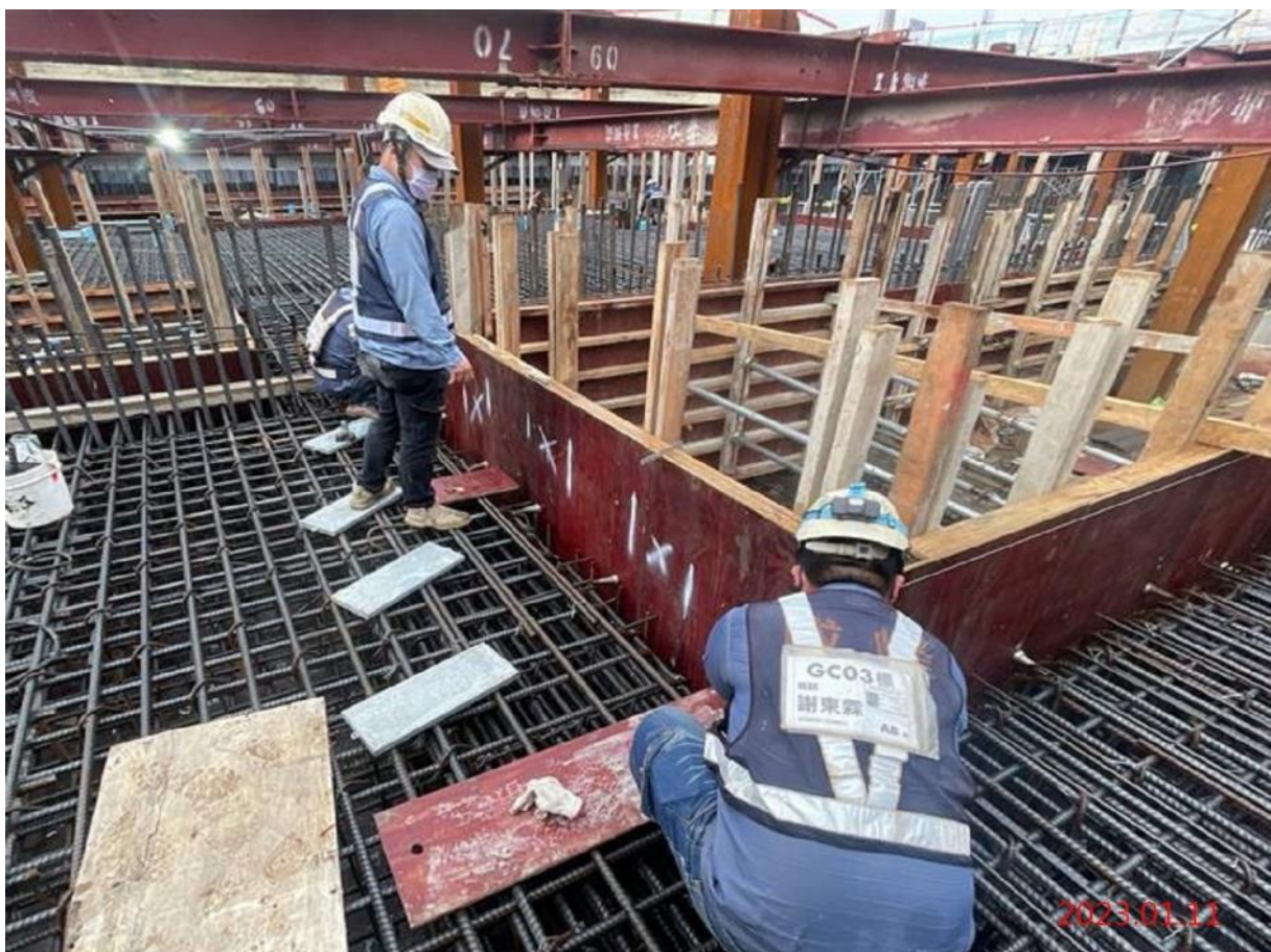
G12 站_出入口夾層版模板組立
