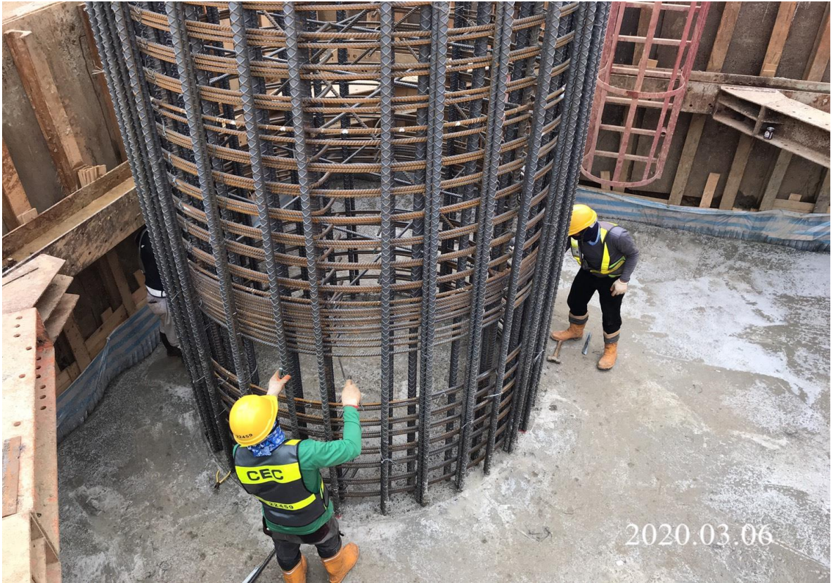
蘆竹中正北路 墩柱第一層鋼筋綁紮
