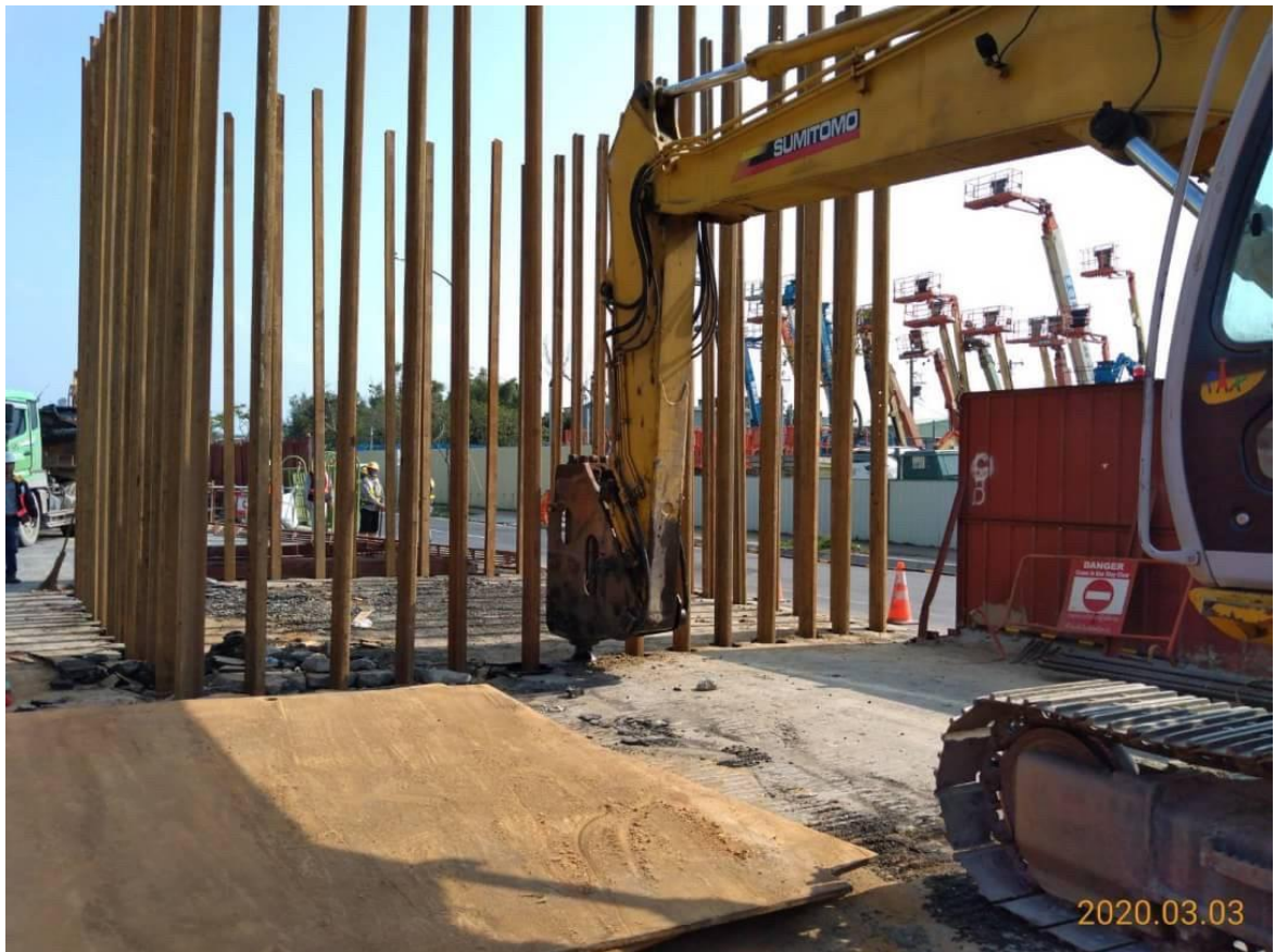
蘆竹中正北路 樁帽鋼軌樁打設
