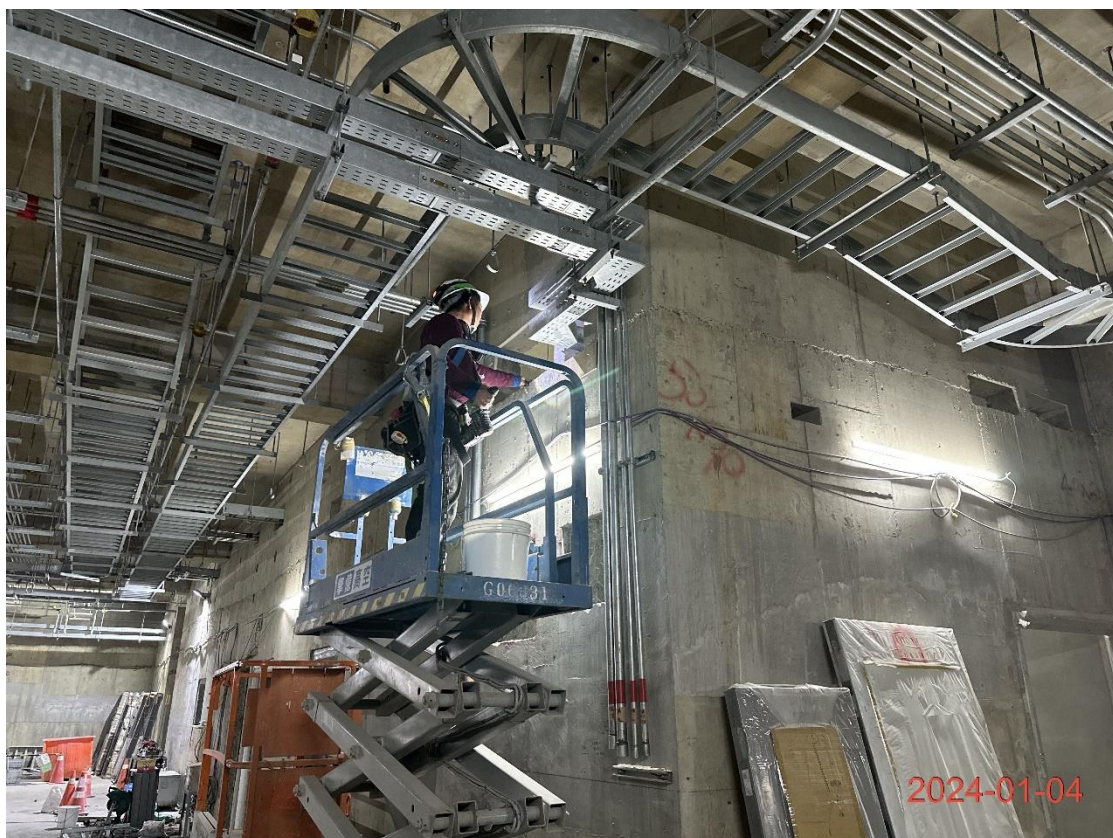
G13 站通訊系統線槽配管施作
