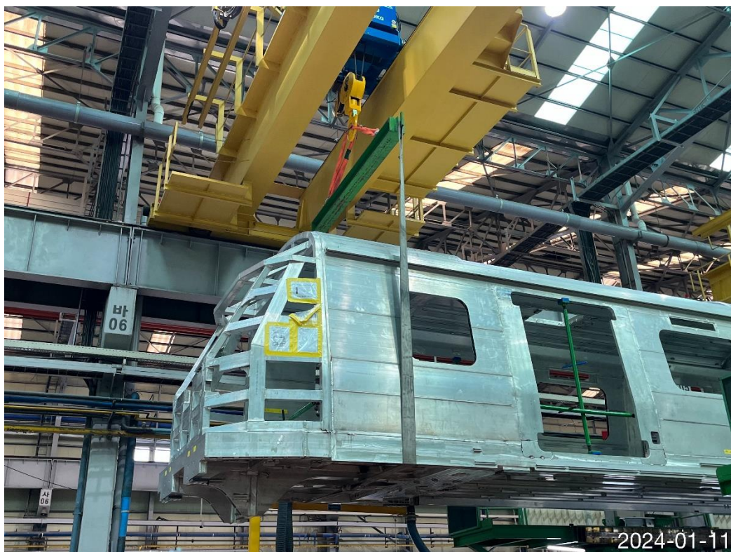
捷運綠線首列車廂於韓國昌原工廠完成焊接及組立
