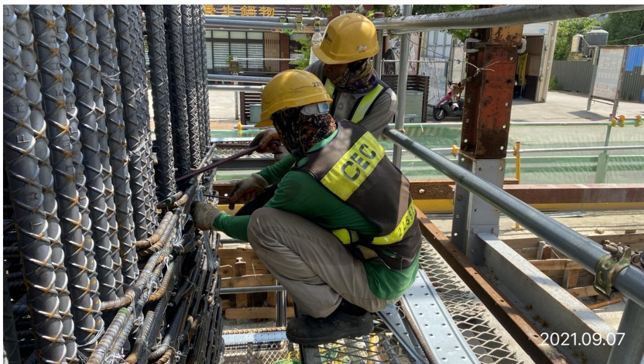
蘆竹中正北路 墩柱鋼筋綁紮
