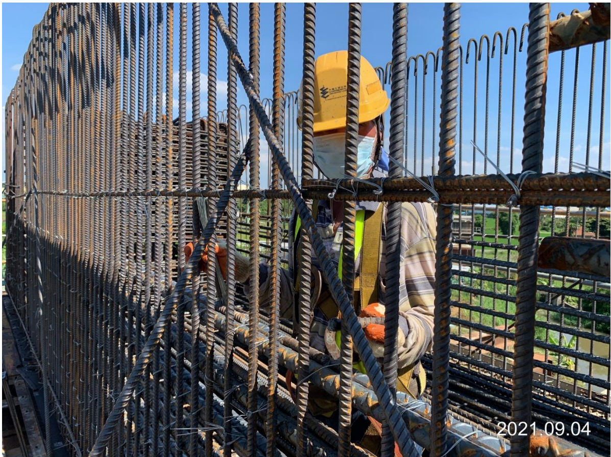
八德新闢道路 帽梁鋼筋綁紮
