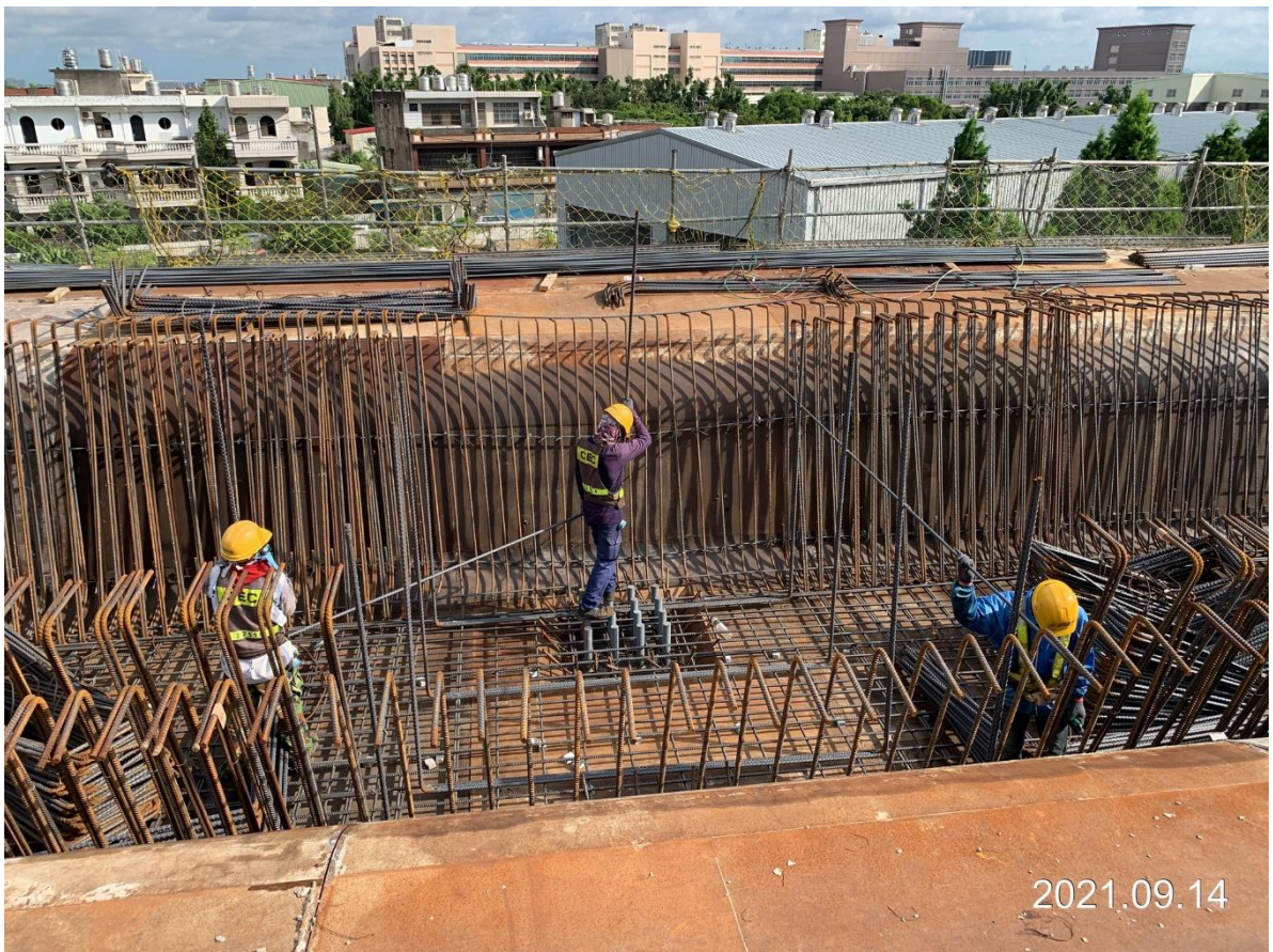
八德新闢道路 場鑄箱型梁底腹版鋼筋綁紮
