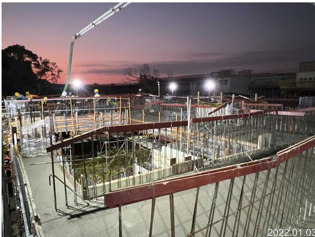
八德新闢道路 G02 車站出入口混凝土澆置
