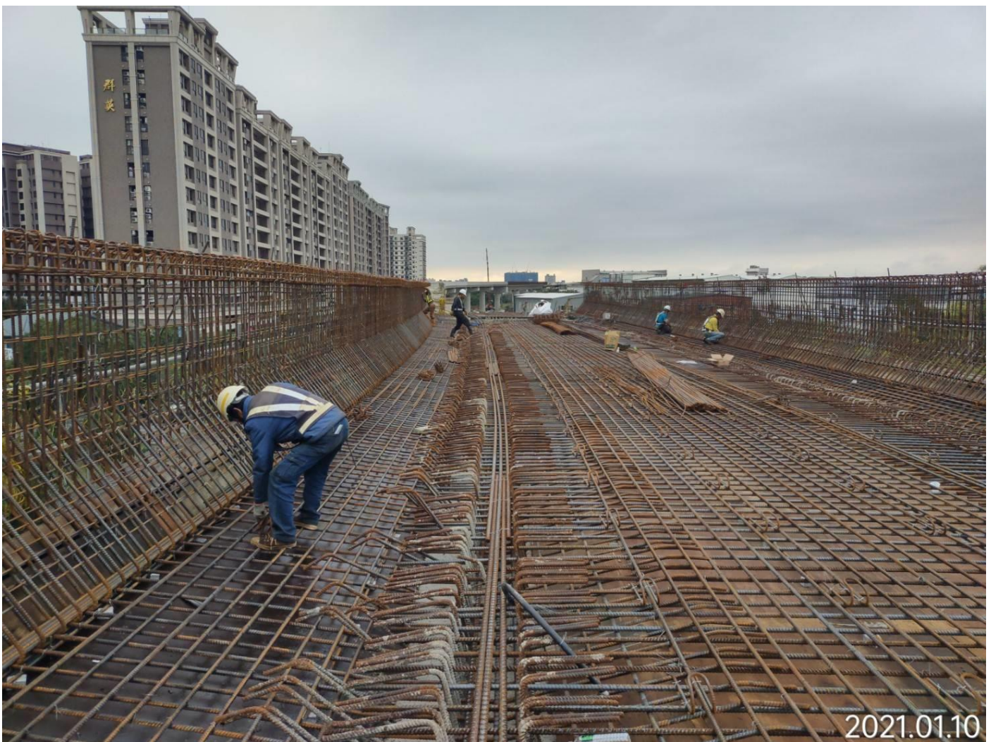
八德新闢道路 場鑄箱型梁鋼筋綁紮
