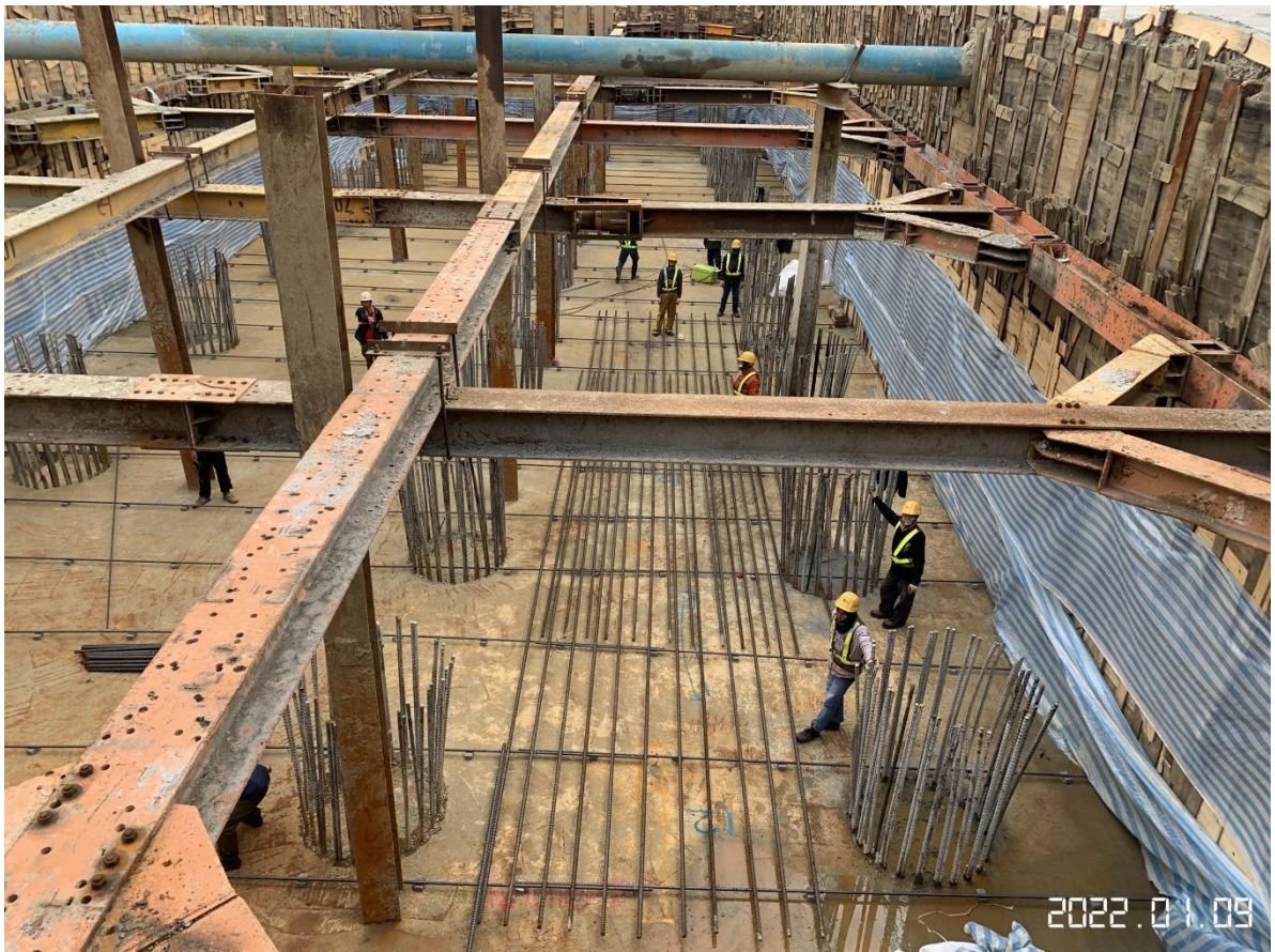
大園坑菓路 樁帽鋼筋綁紮
