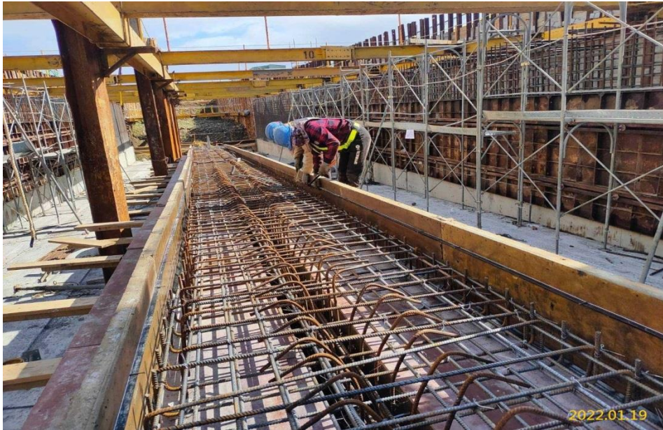
南出土結構體鋼筋綁紮
