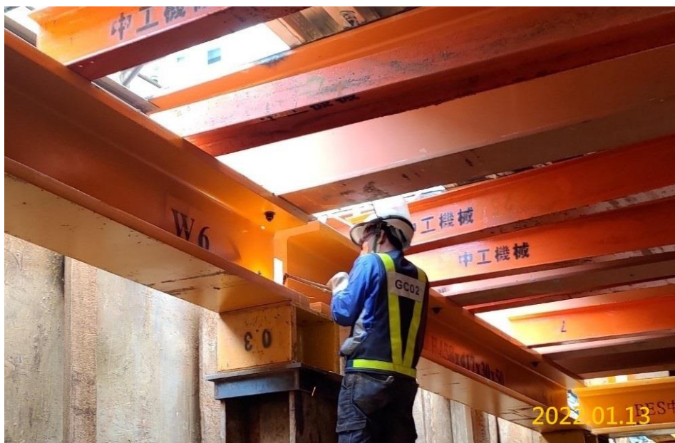
G06 站覆蓋系統施作
