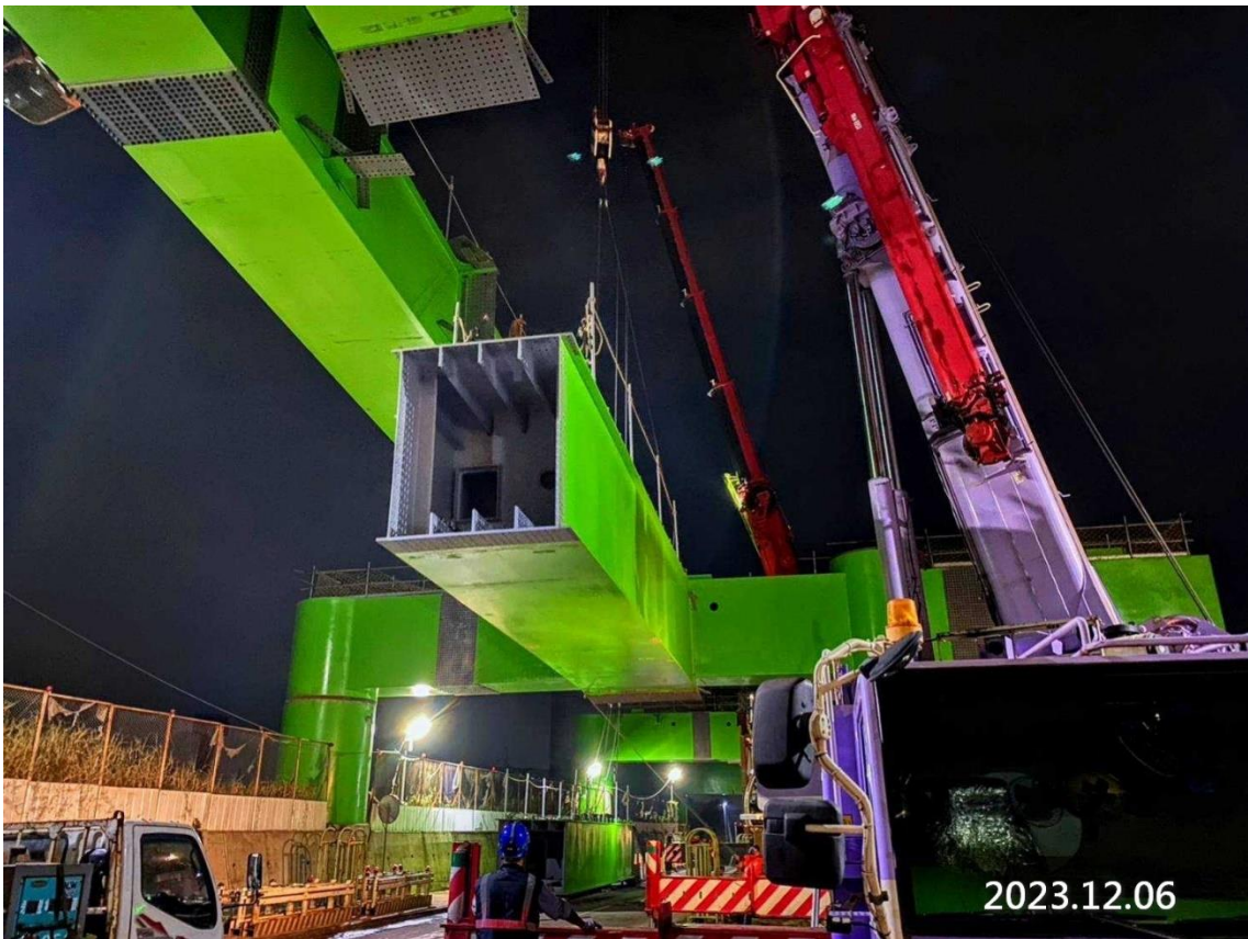
DU14-06 鋼箱樑(B06、B07)進料吊裝
