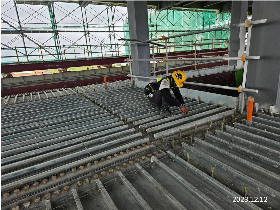
G13a 站體月台層 Deck 版鋼筋與點焊鋼絲網吊運
