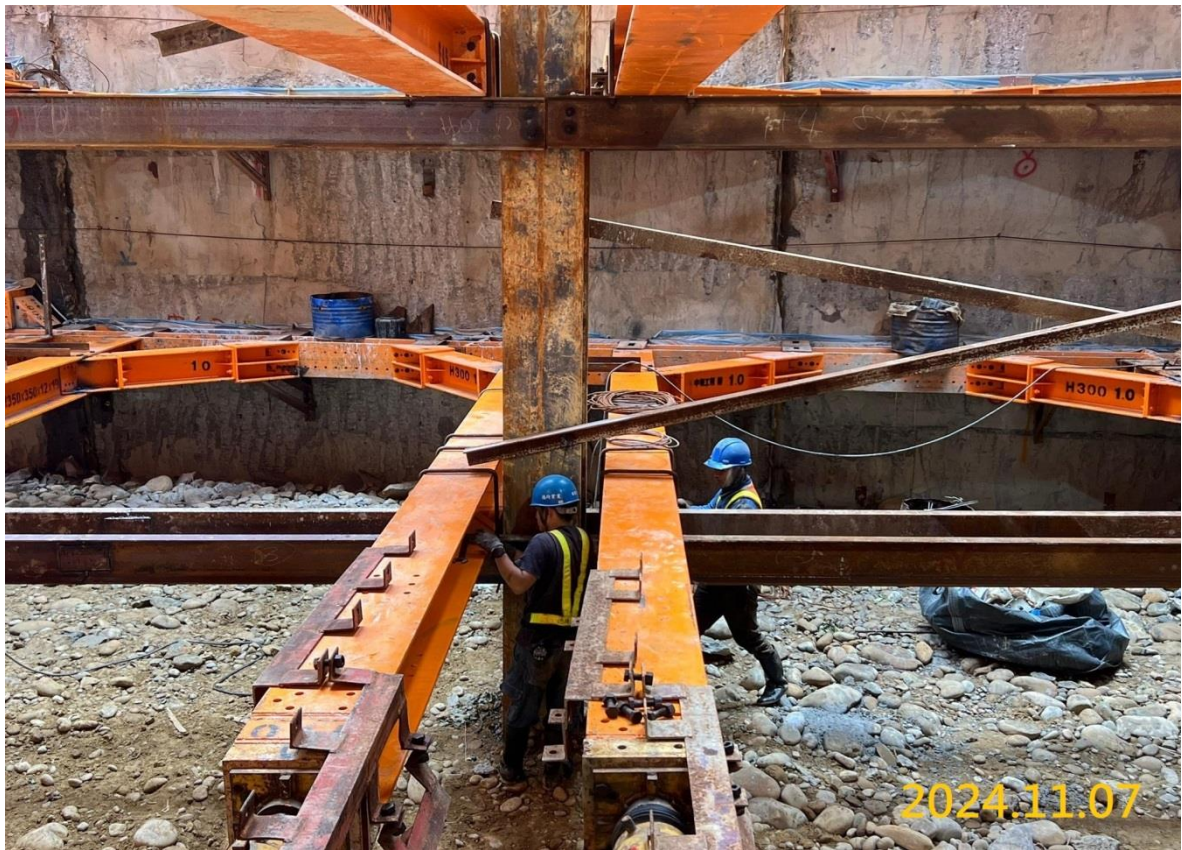
維修軌明挖覆蓋段支撐架設
