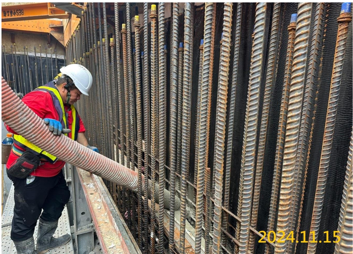
G06 出入口結構牆施作
