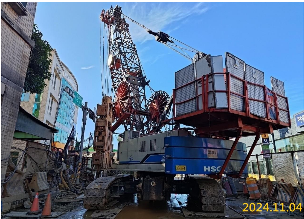
G04 站連續壁施作
