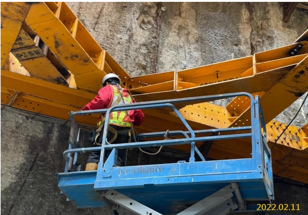
VS6 通風豎井支撐系統拆除
