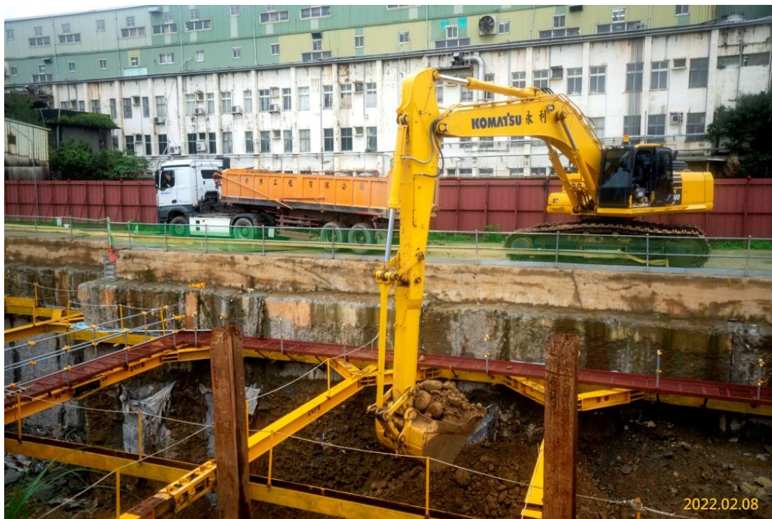
南出土結構體開挖施作
