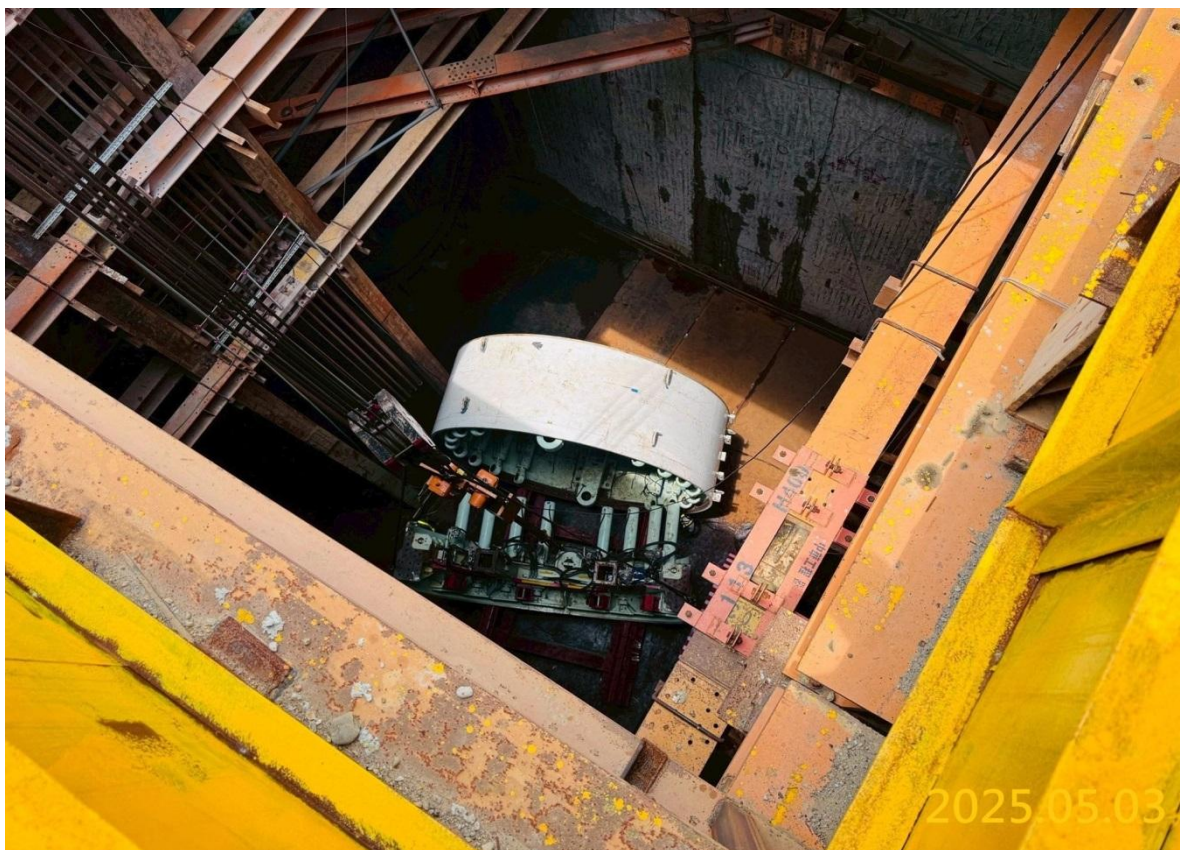
G06 站潛盾隧道發進前置作業-潛盾機組裝
