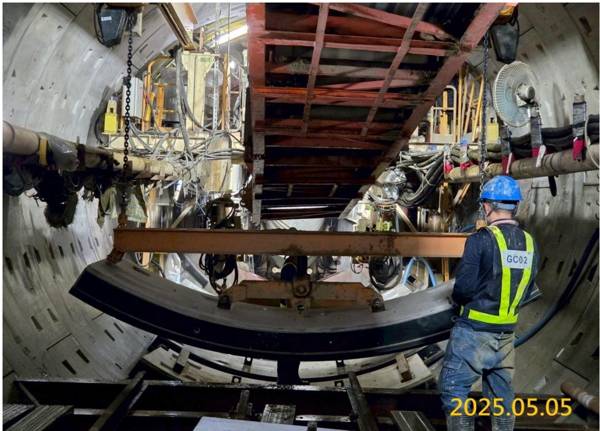
G03 站南井潛盾隧道掘進施作
