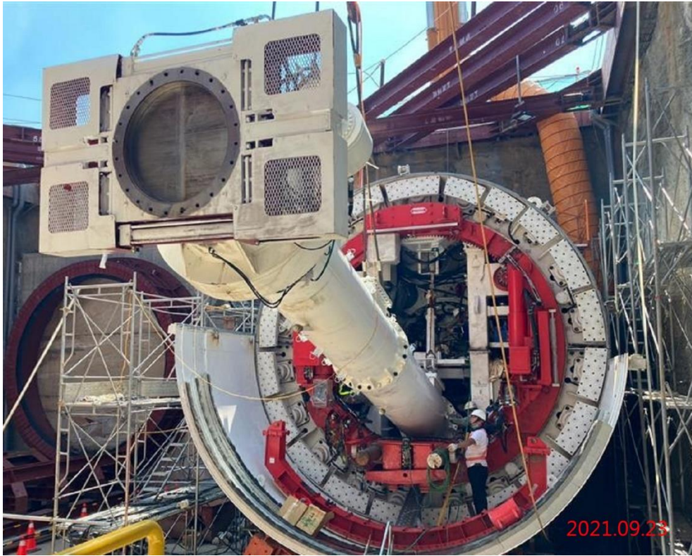
北出土段_潛盾隧道_潛盾機組裝
