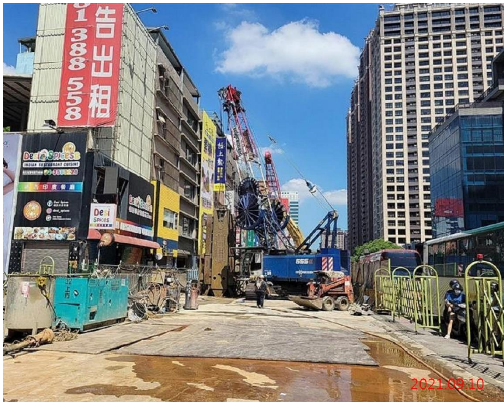
G10 站_連續壁單元挖掘
