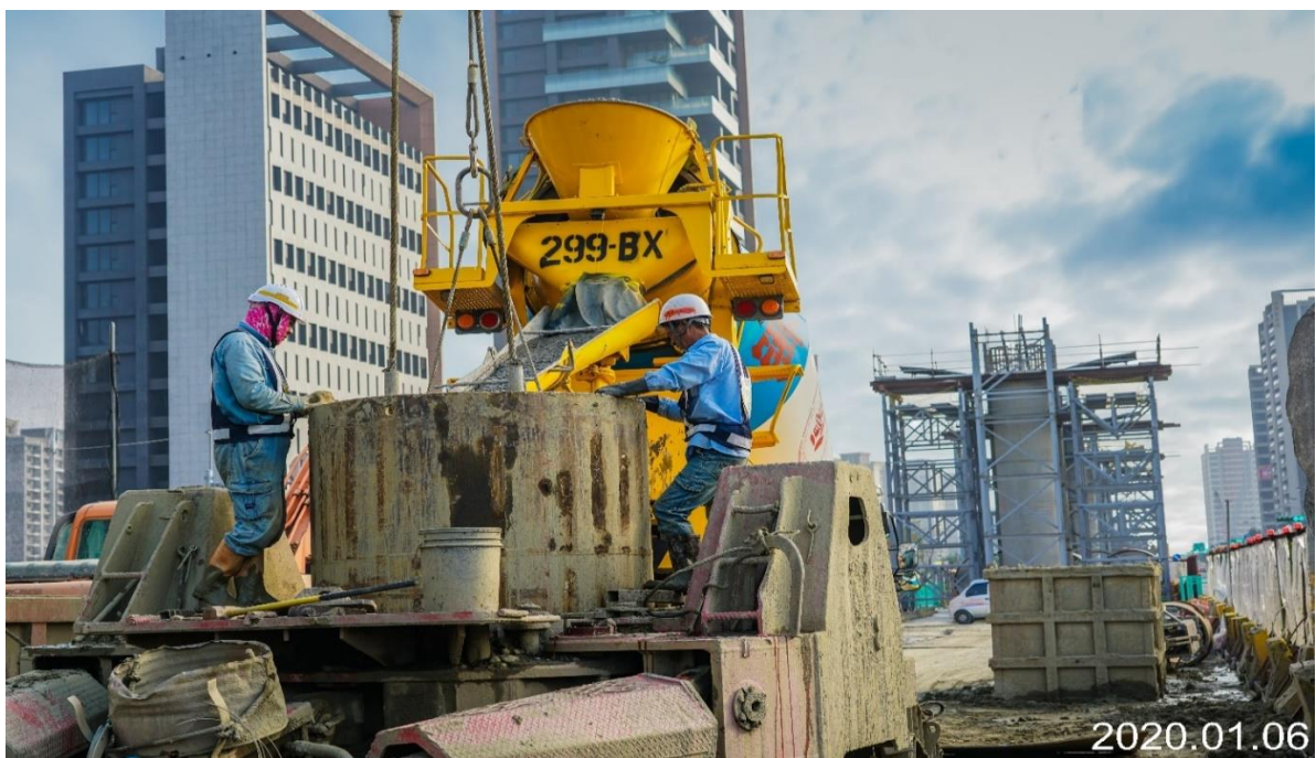
八德建德路 基樁混凝土澆置
