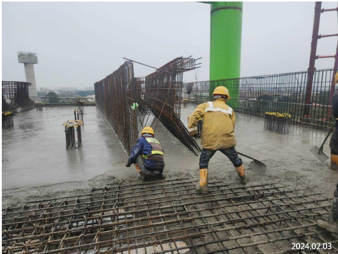
北段上構_DU14-06 下行線橋面版混凝土澆置
