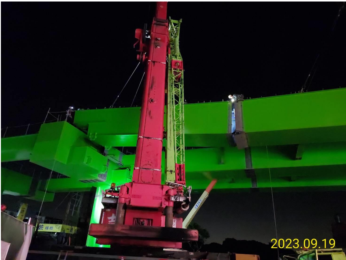
鋼構 DU14-01 鋼箱梁(C01 ~ C02)起吊接合
