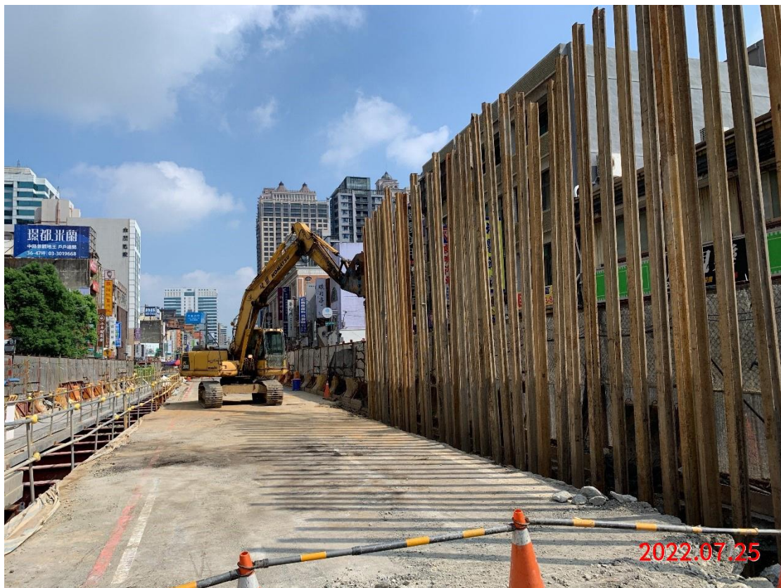
G10 站_工作井鋼軌樁打設
