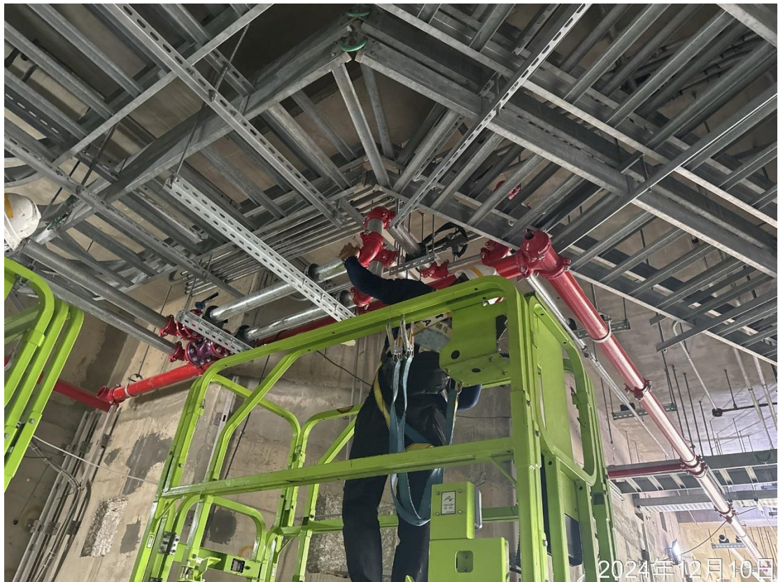
G13a 站 3F 空調系統配管
