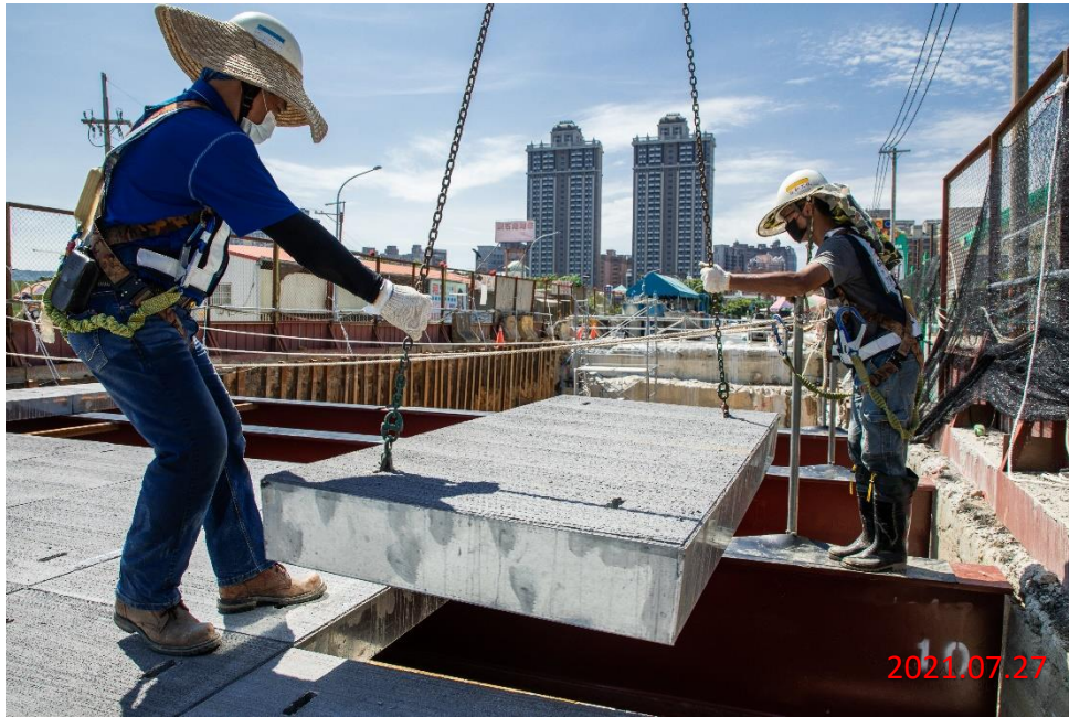
G12 站_覆工版樑安裝作業
