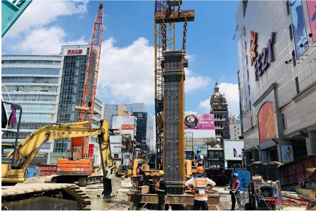
G07 站_逆打鋼柱吊放作業
