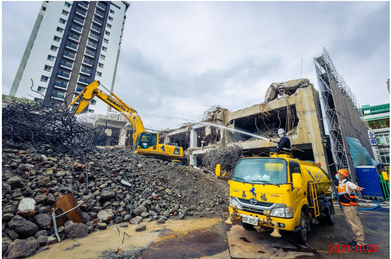
G08 站_結構拆除作業
