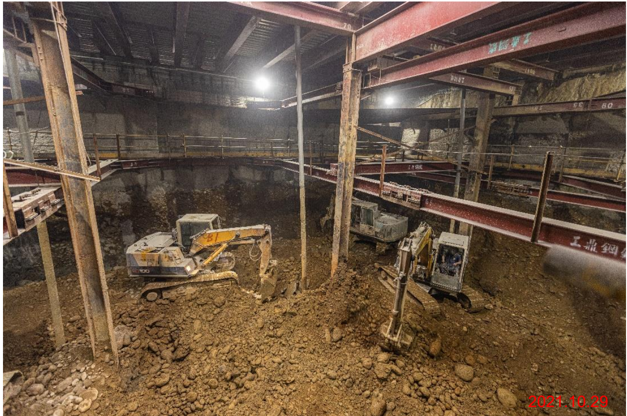
G12 站_站體第三撐開挖施作
