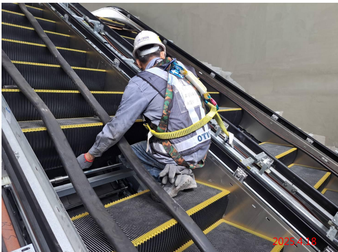
G12 站 1-2 號電扶梯踏階安裝作業
