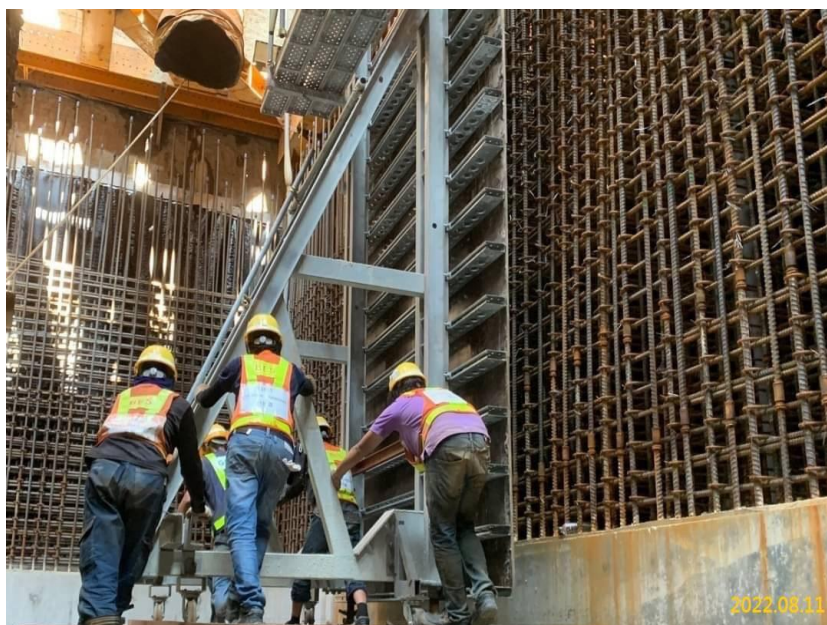
VS6 通風豎井結構體系統模板組立
