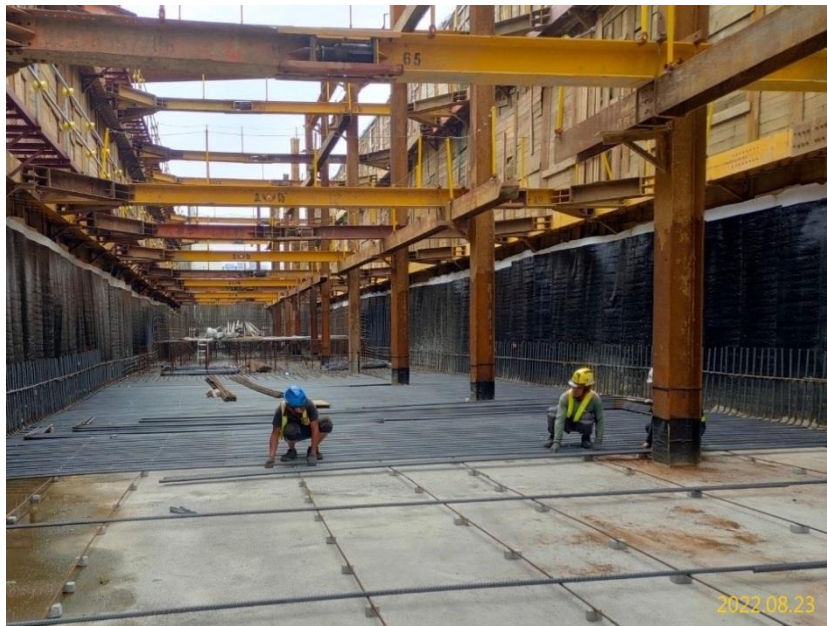
南出土段底版施作
