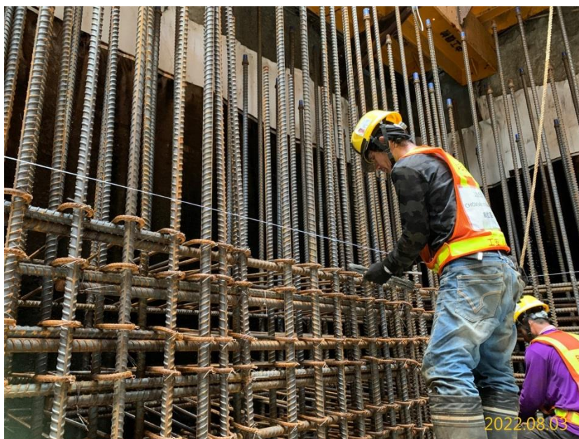
VS6 通風豎井結構體鋼筋綁紮
