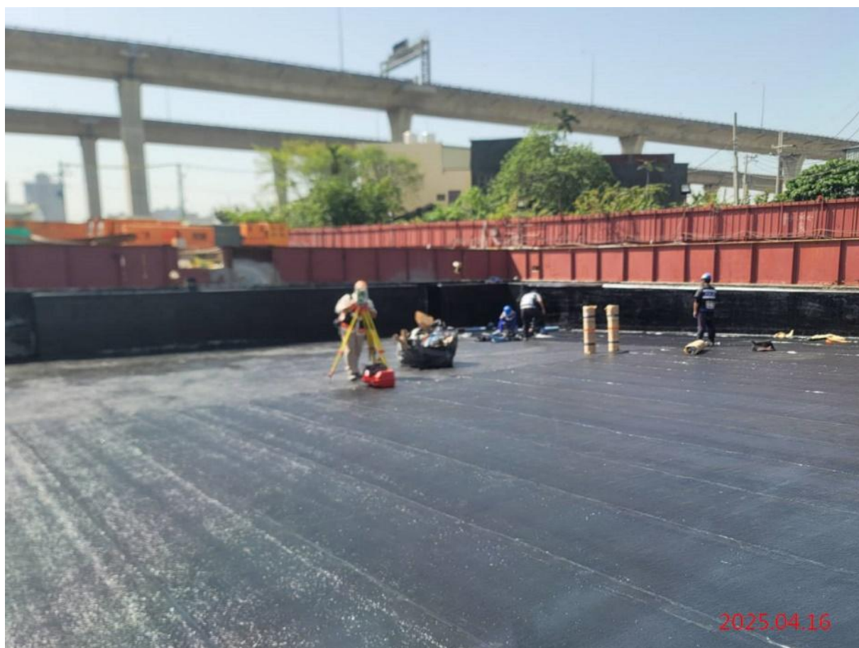
北出土段_頂版防水膜施作
