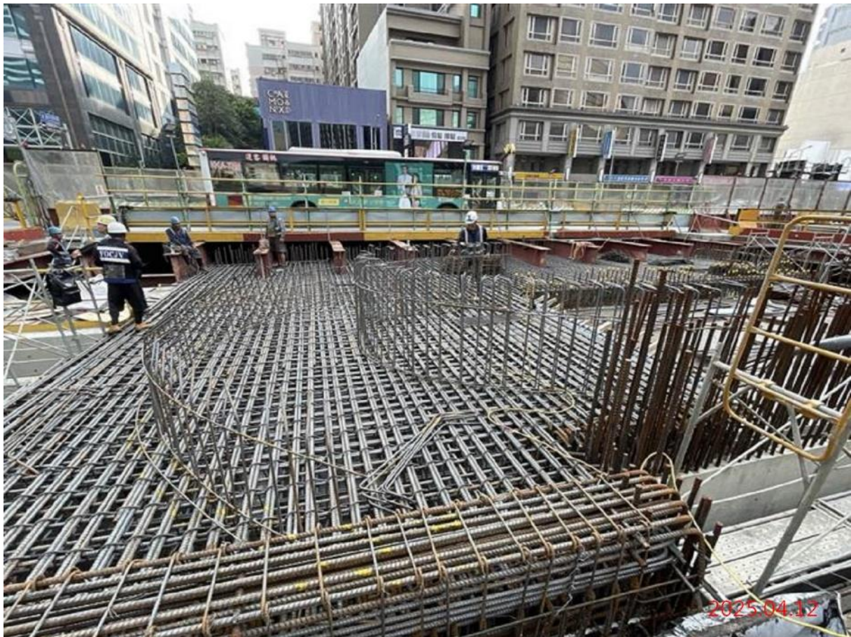
G11_出入口 B 地面層頂版鋼筋施作
