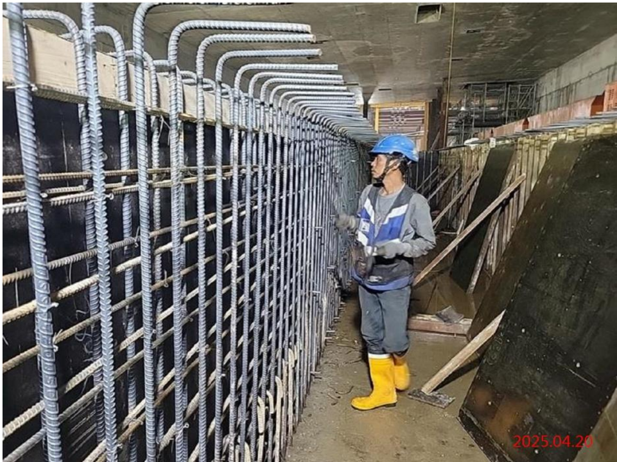
G10_站體軌道層月台版模板組立
