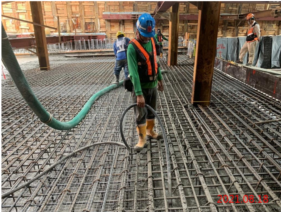
北出土段_底版混凝土澆置
