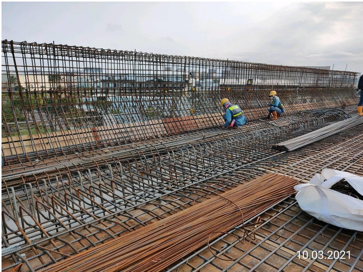
八德新闢道路 場鑄箱型梁橋面版鋼筋綁紮
