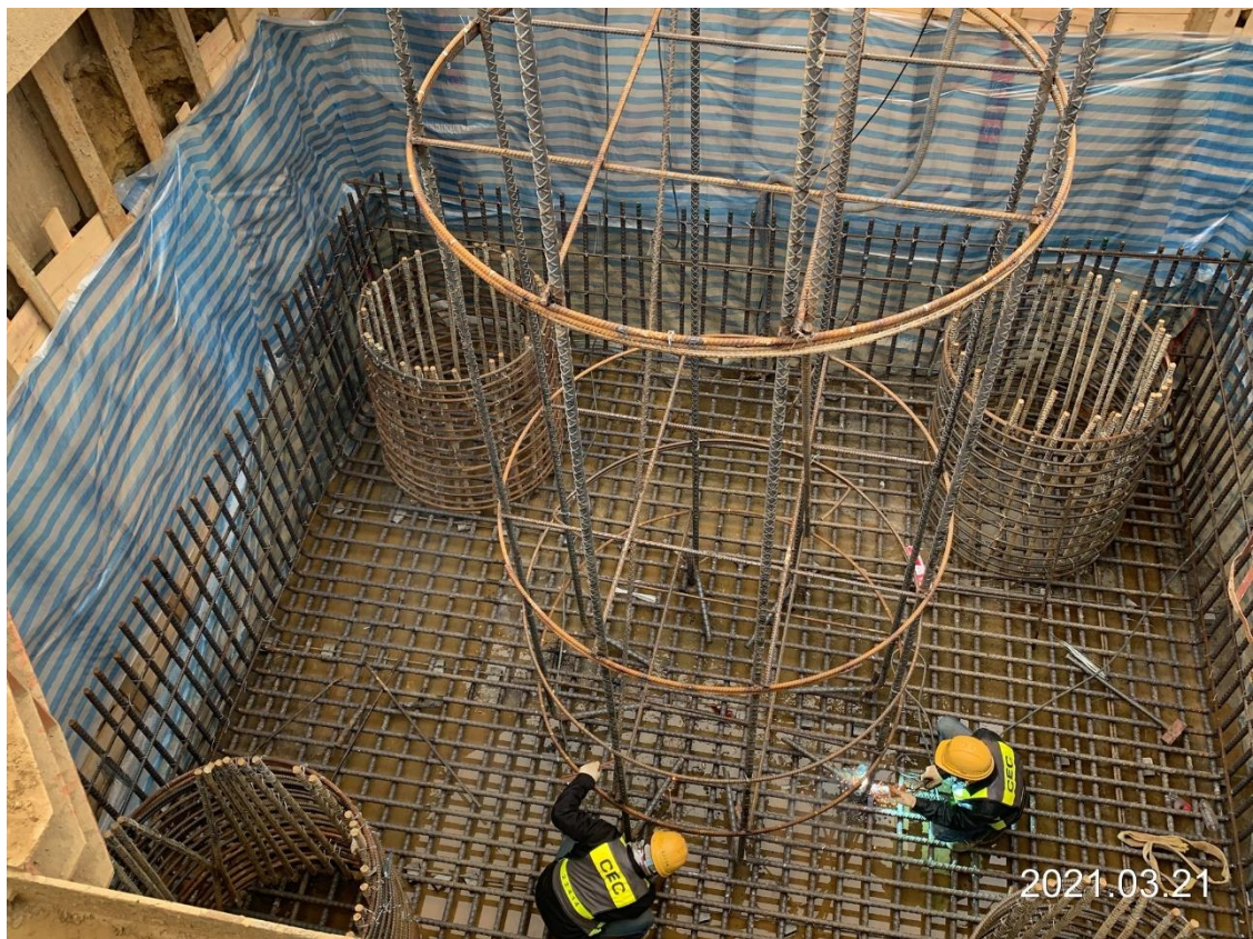
八德新闢道路 樁帽鋼筋綁紮
