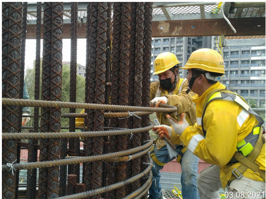
八德新闢道路 墩柱鋼筋綁紮
