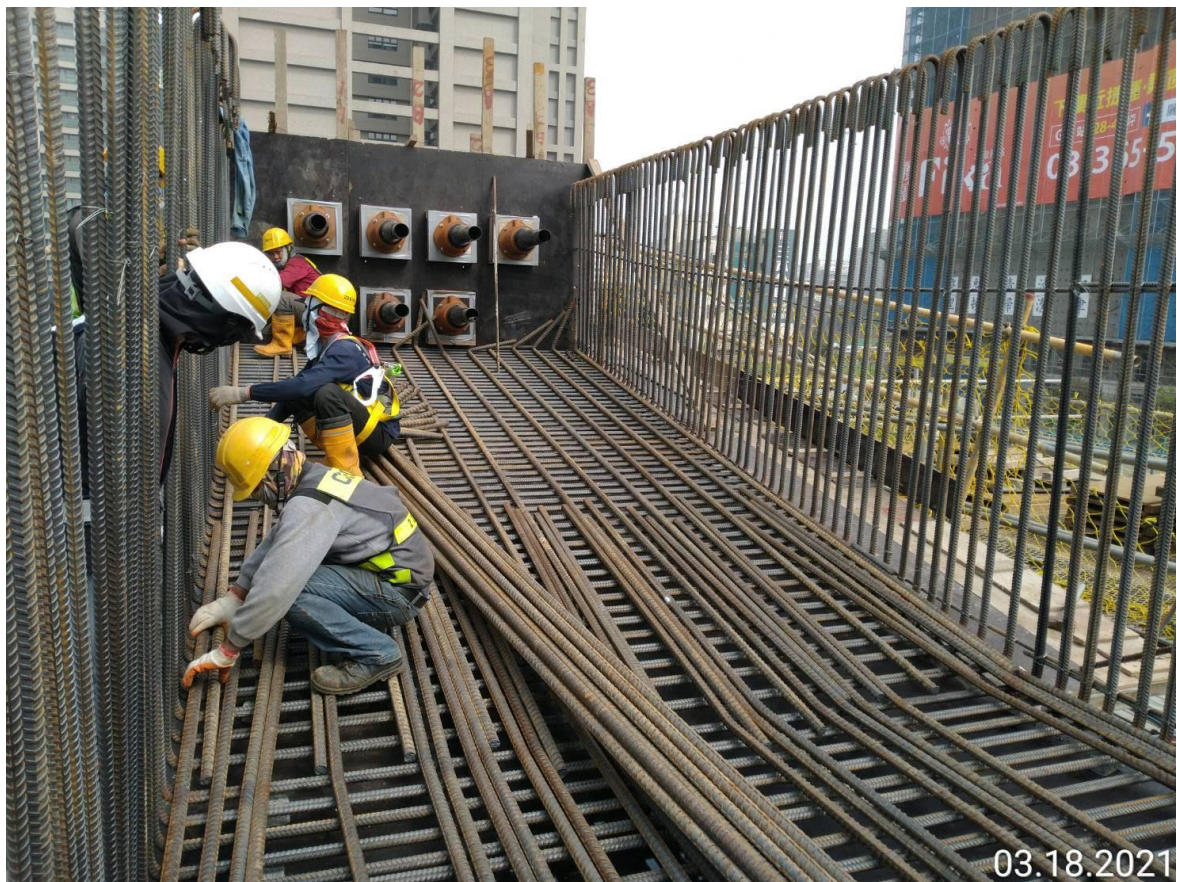
八德建德路 帽梁鋼筋綁紮
