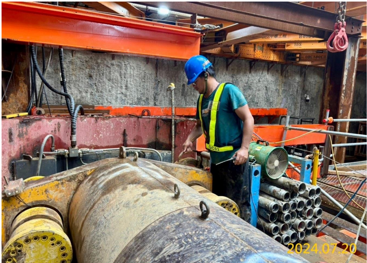
VS4 通風豎井管幕推進
