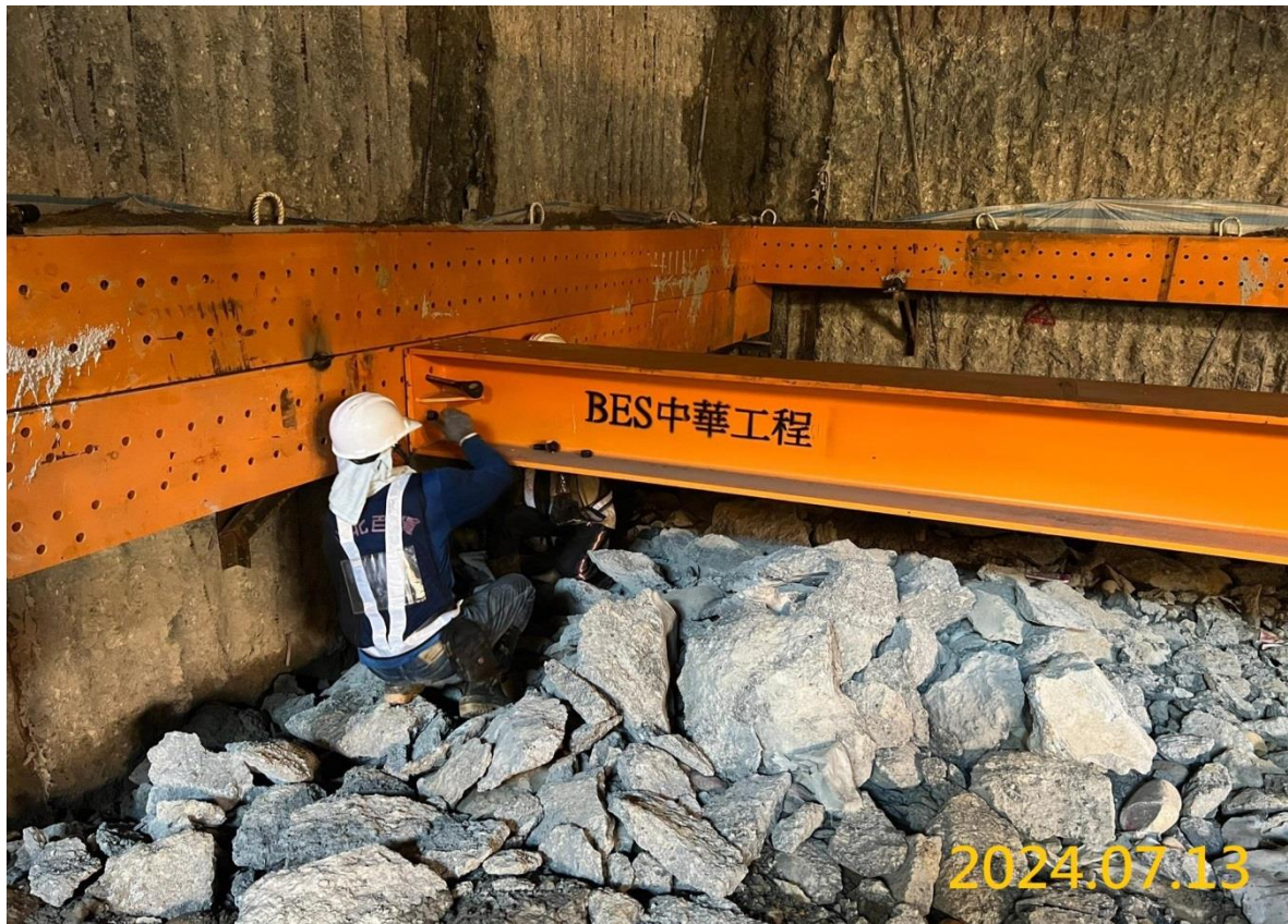
G05 站開挖支撐施作
