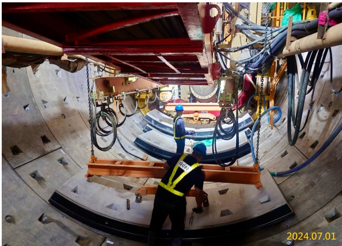
G03 站潛盾隧道掘進施作
