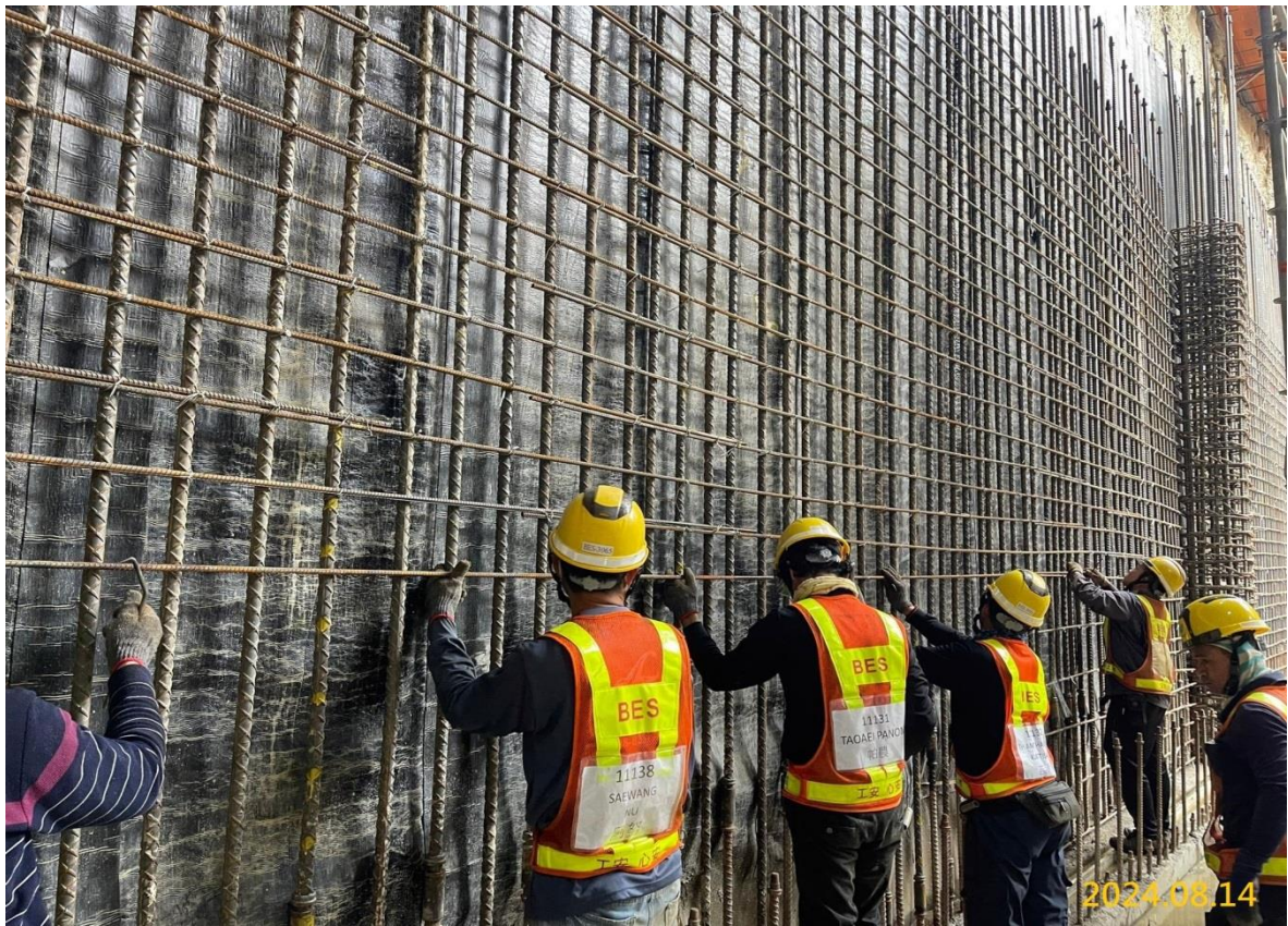
G03 站結構牆施作
