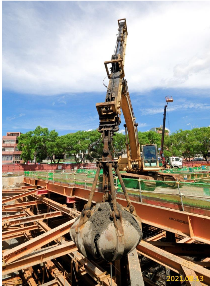
VS6 通風豎井開挖支撐施作
