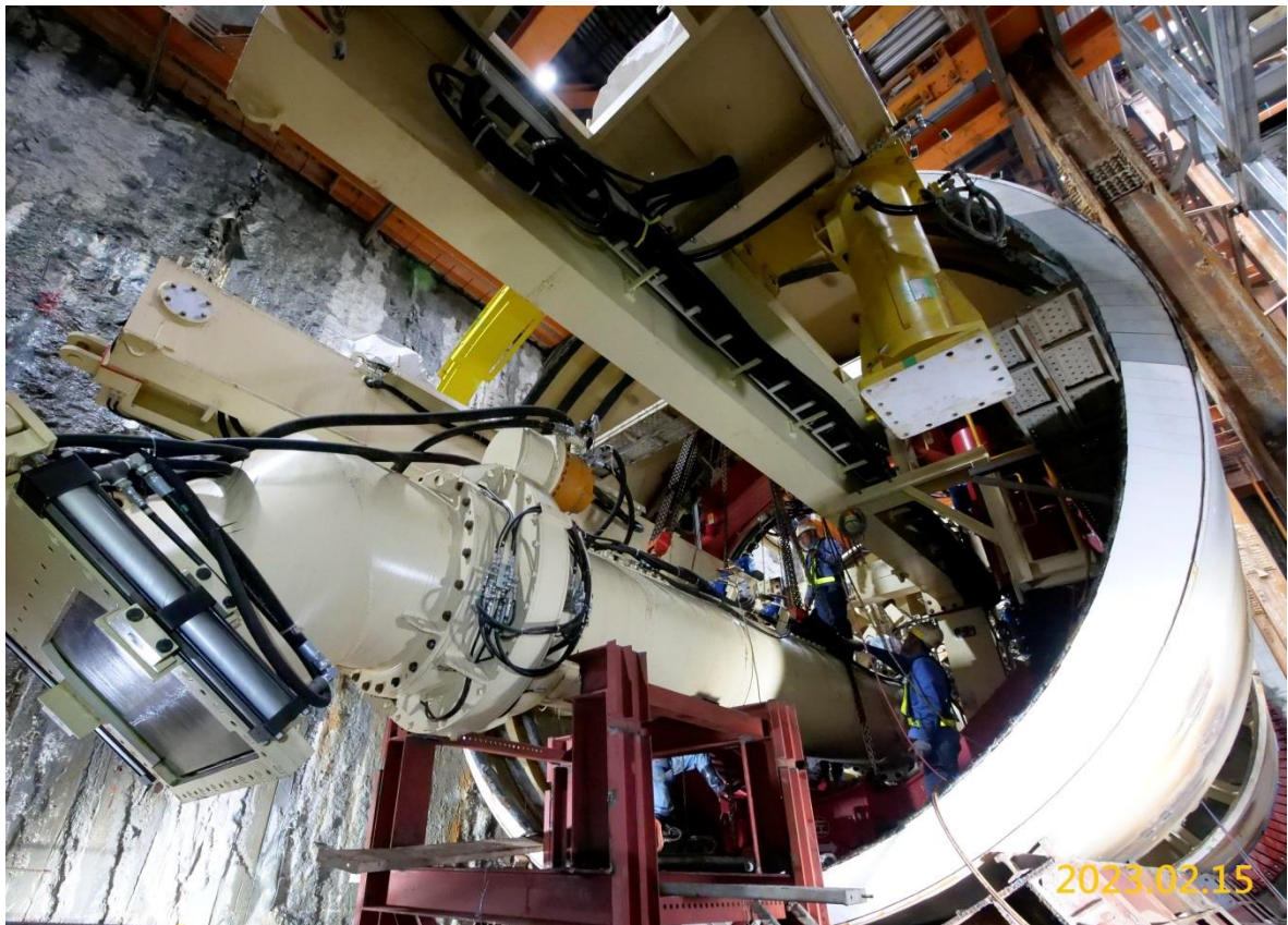
G03 站潛盾機投入組立
