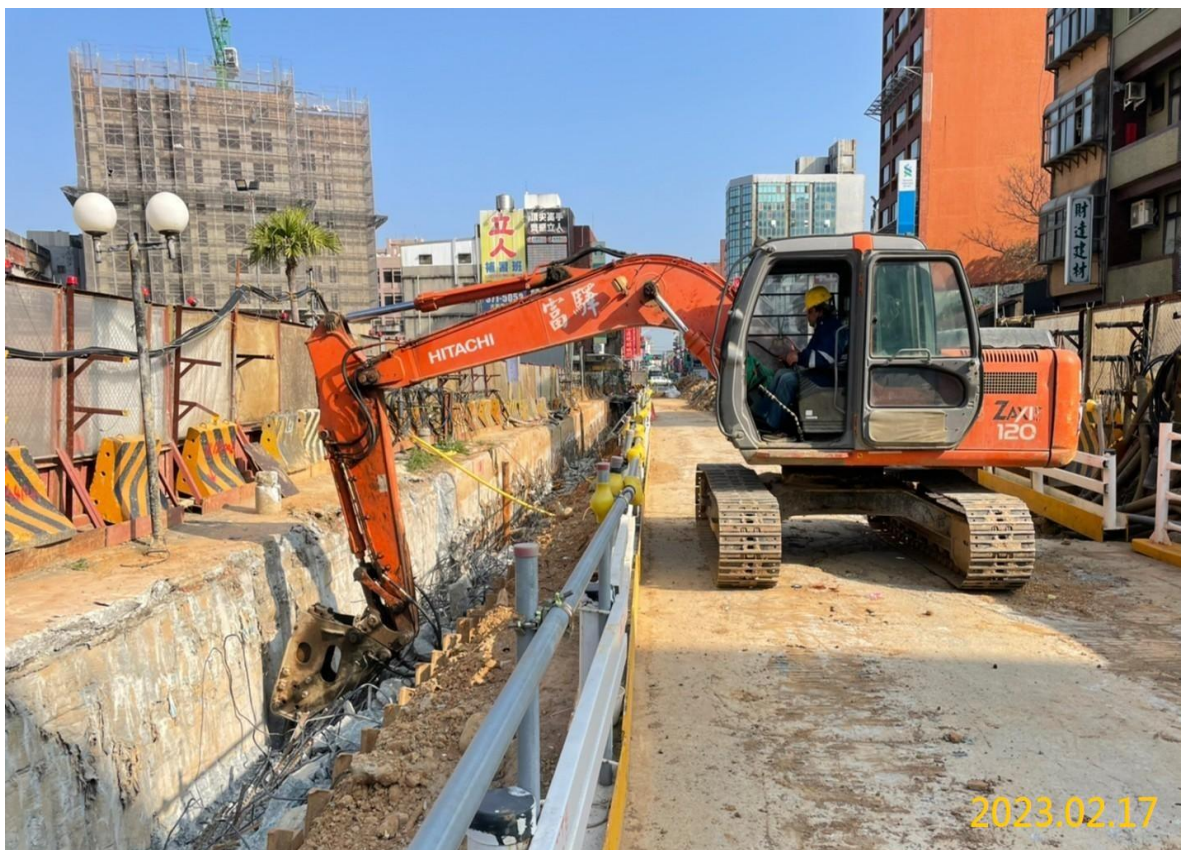
G04 站臨時排水施作
