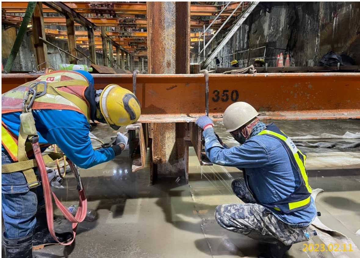
南出土段支撐施作
