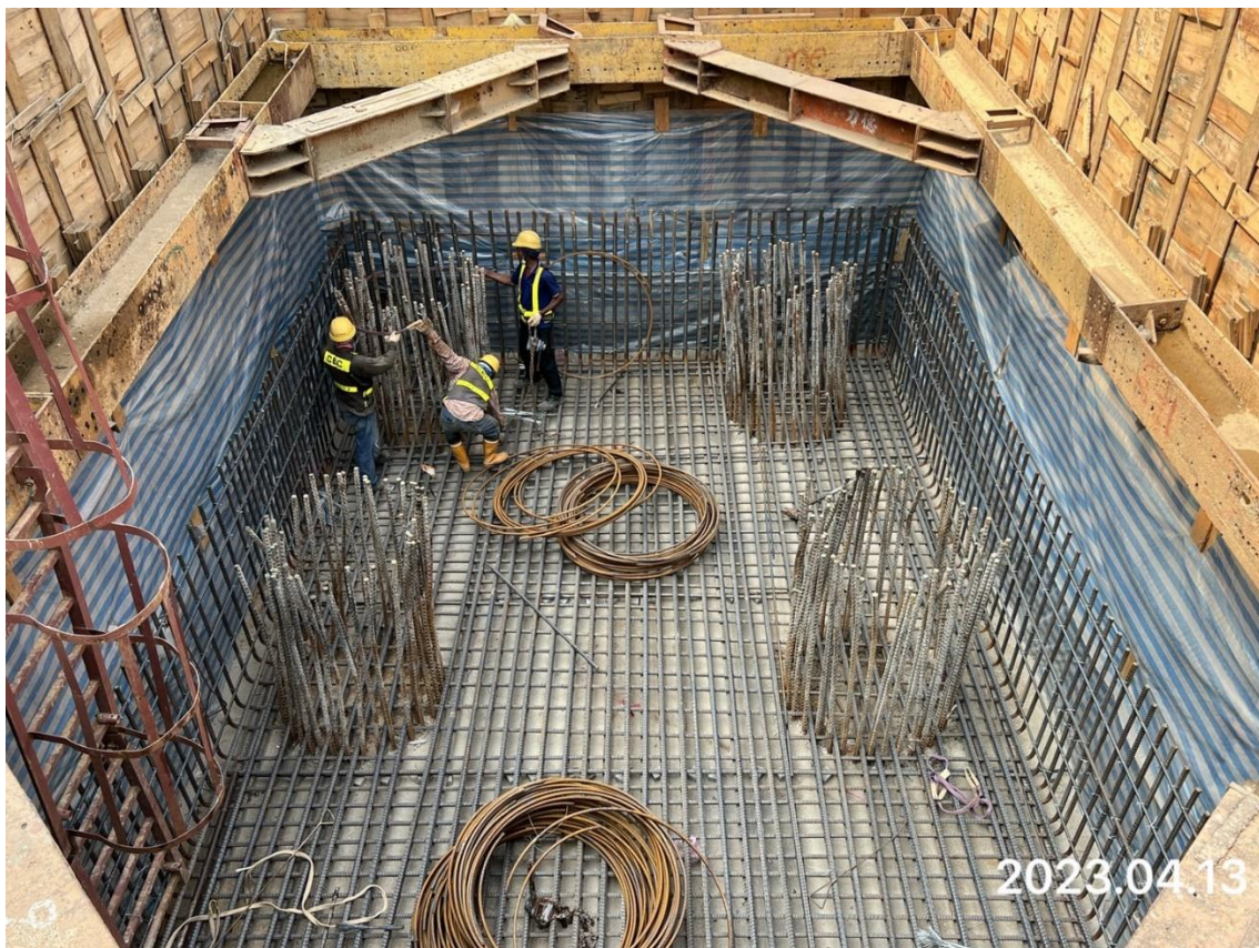
北段_E 工區_樁帽 PD-01 下層筋綁紮
