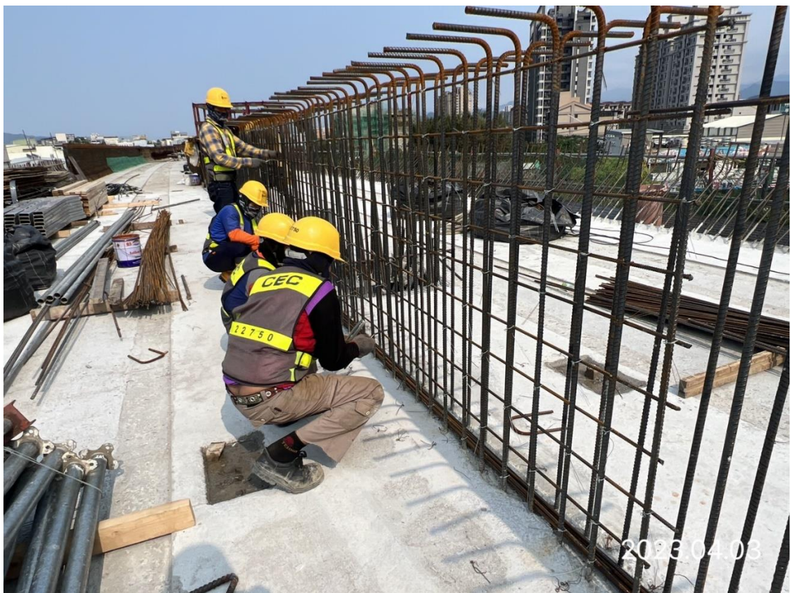
北段上構_DU31-09 中央走道鋼筋綁紮
