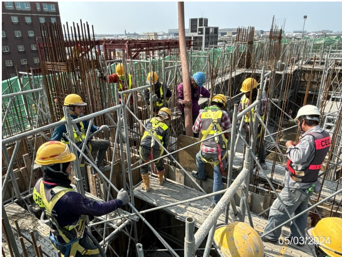
北段_G31 車站出入口四樓柱牆第一昇層混凝土澆置
