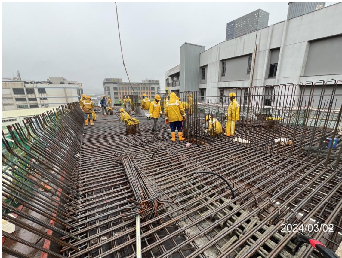
北段上構_DU13a-09-3 場撐箱型梁頂版鋼筋綁紮
