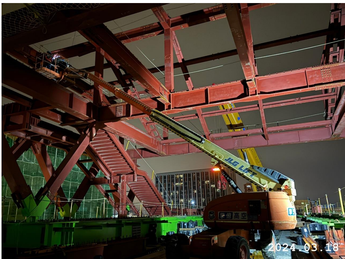
鋼構組_G31 站體螺栓穿鎖作業
