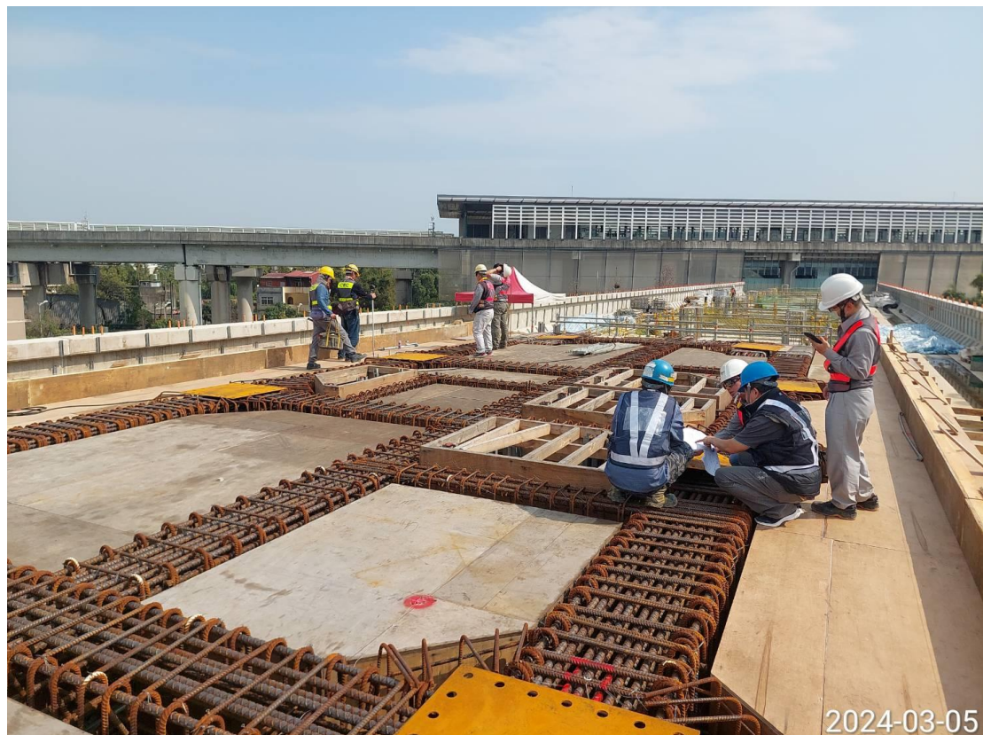
北段上構_G32 站月台梁(TG7 ~ TG8)支撐架位置高程檢測
