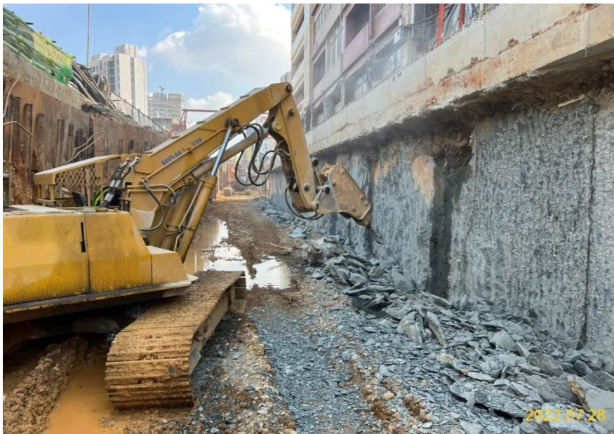
G05 站連續壁面修飾作業
