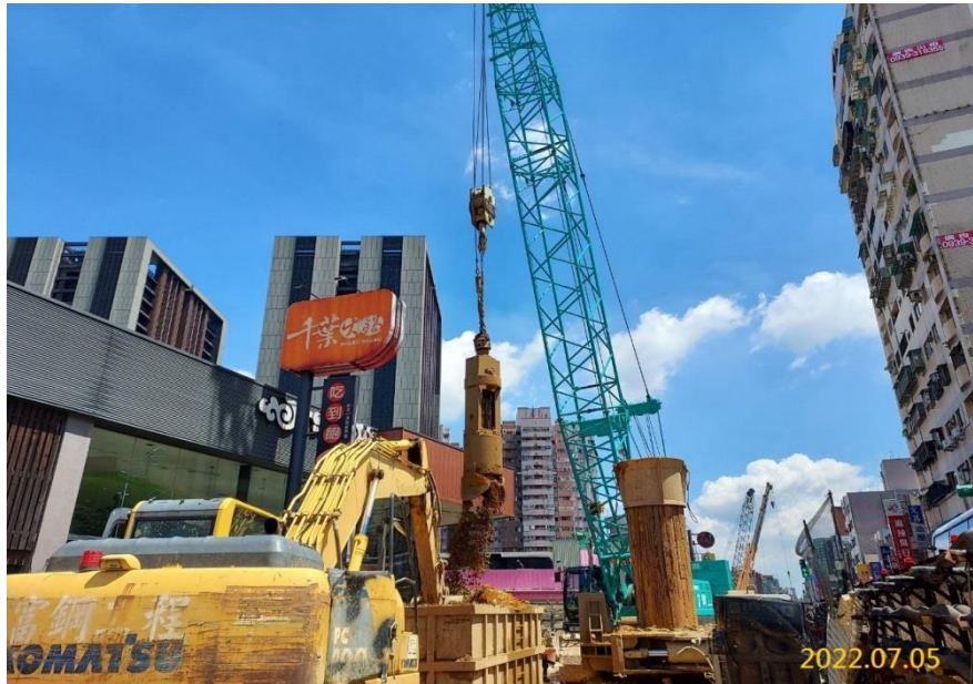
G04 站中間柱施作
