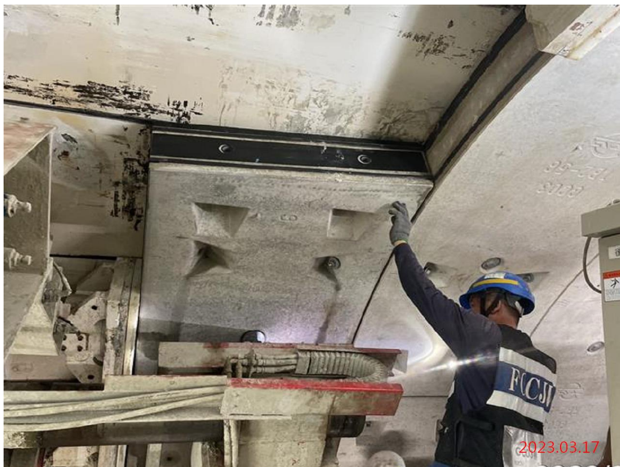
潛盾隧道_小圓環片組立
