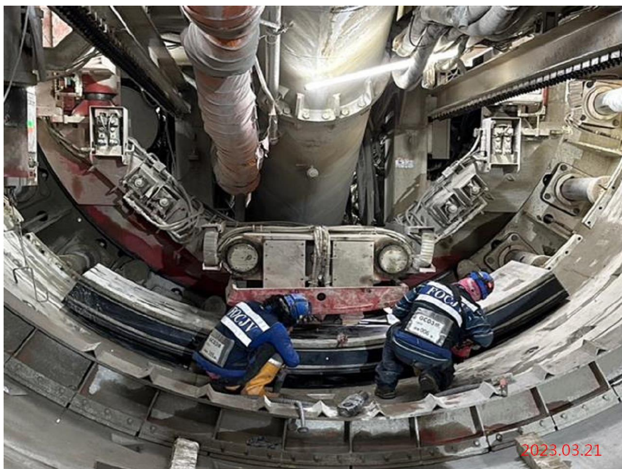
潛盾隧道_小圓潛盾掘進
