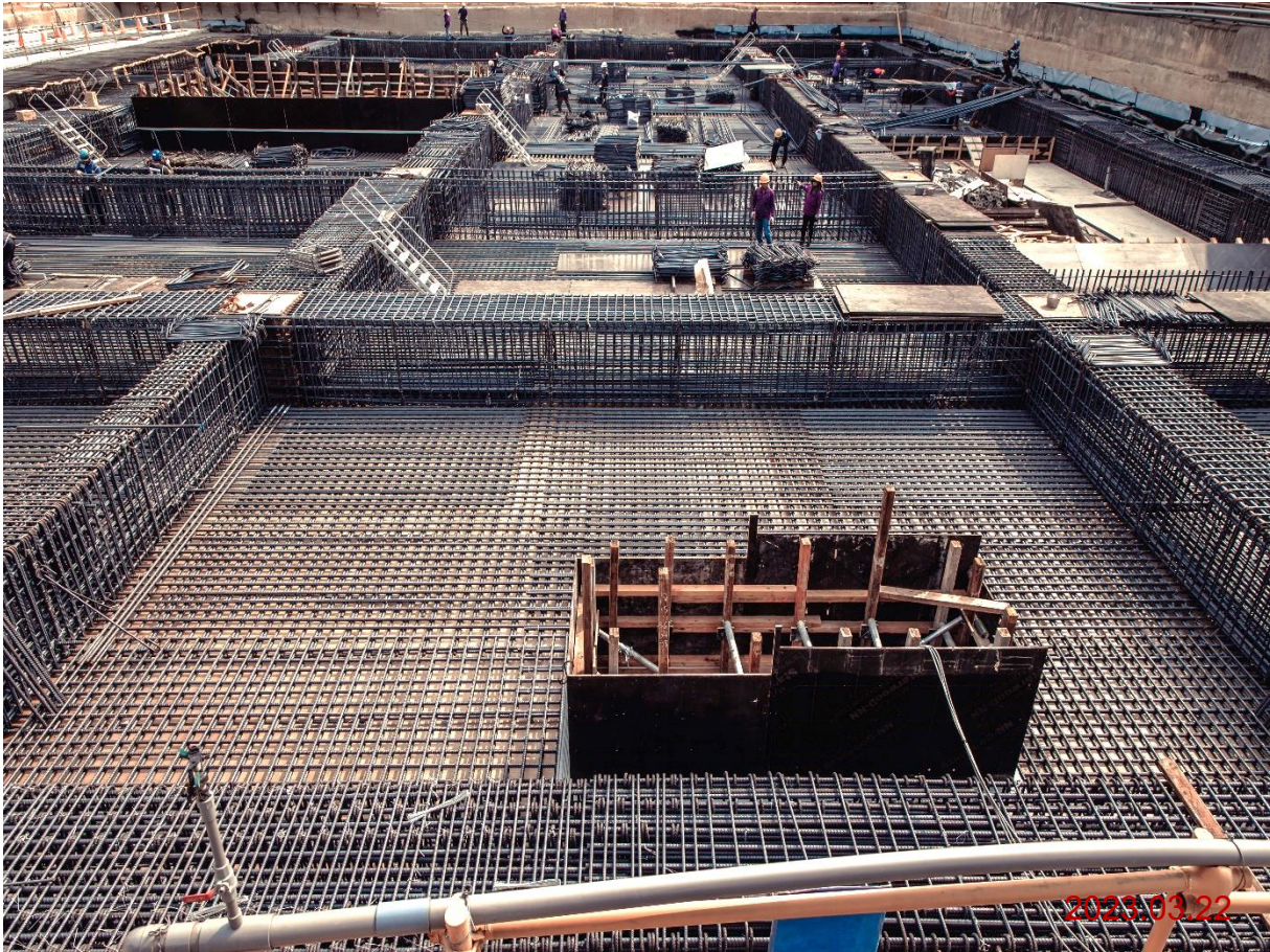
G07 站_站體結構 1FL 版鋼筋綁紮
