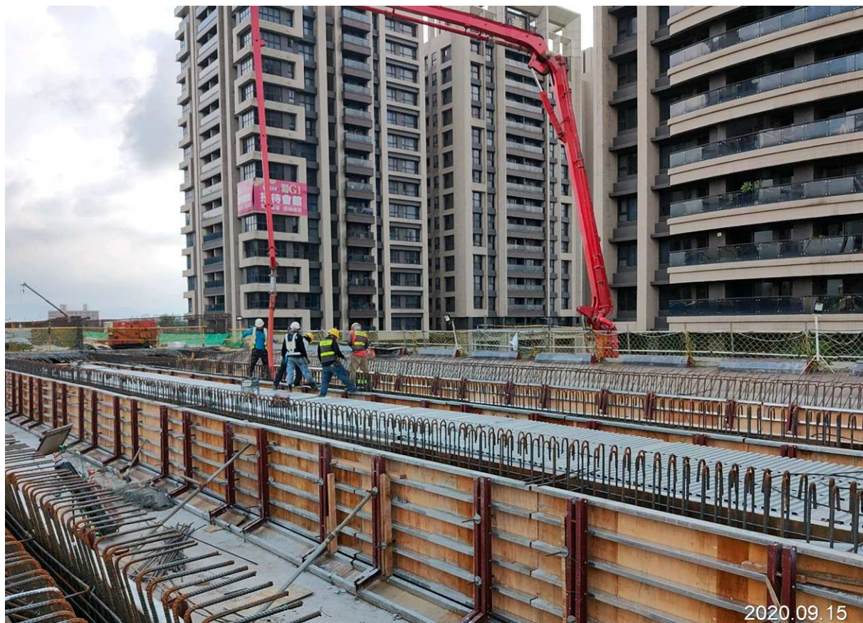
八德建德路 橋面版混凝土澆置
