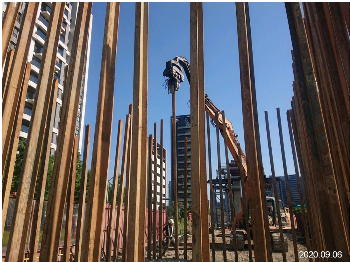
八德新闢道路 樁帽鋼軌樁打設
