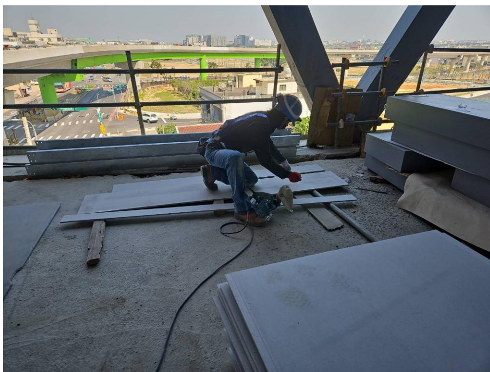
G15a(原 G31)車站站體連通道輕隔間封板
