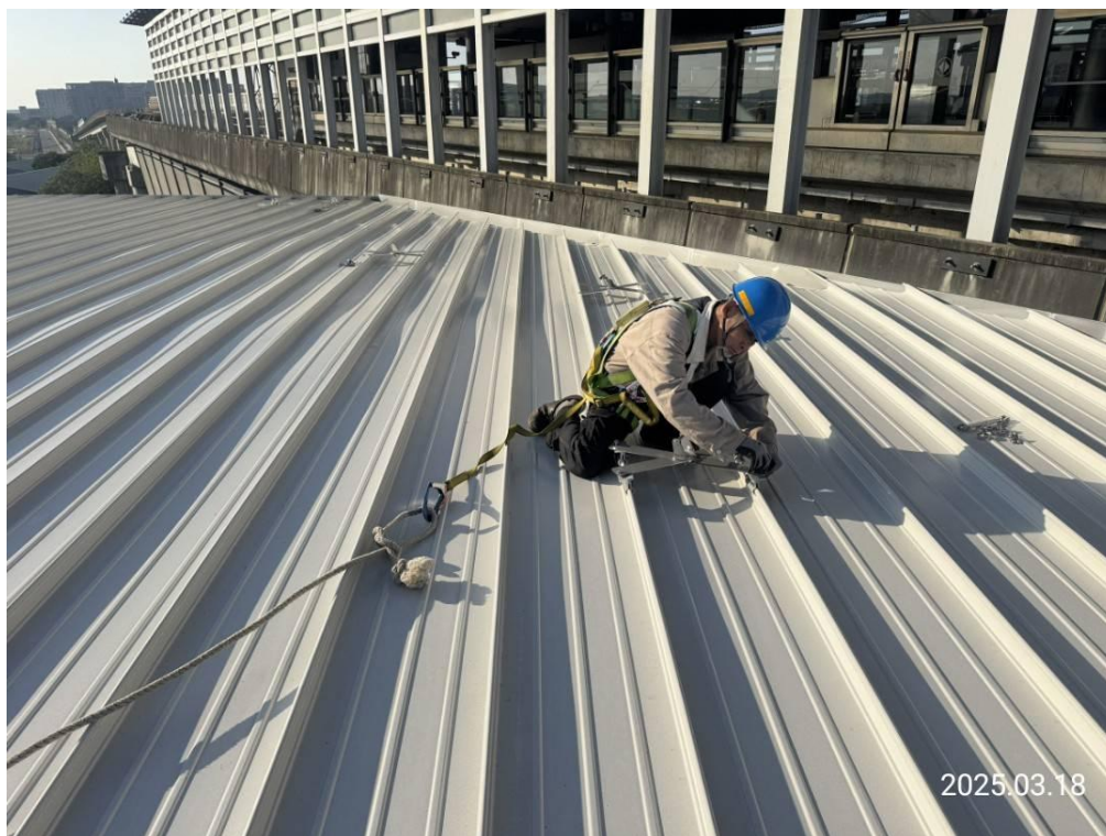
G15b(原 G32)車站站體金屬屋頂防墜系統安裝
