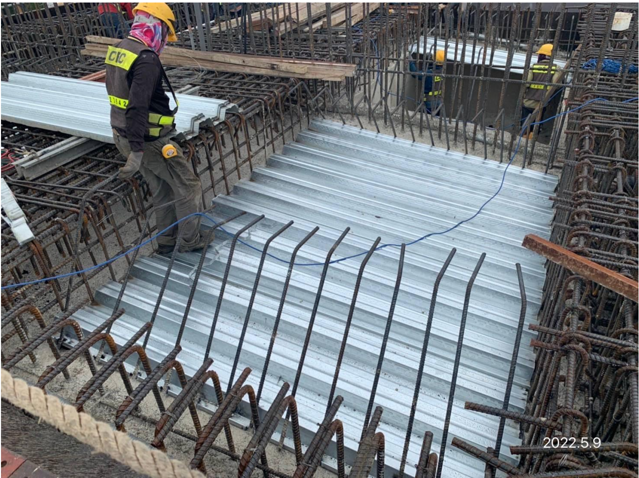
八德新關道路 帽梁模板組立
