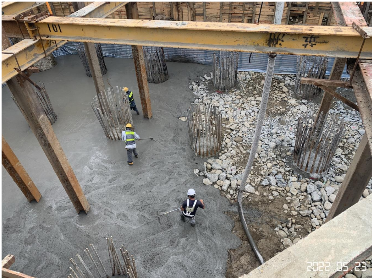
大園坑菓路 樁帽 PC 澆置
