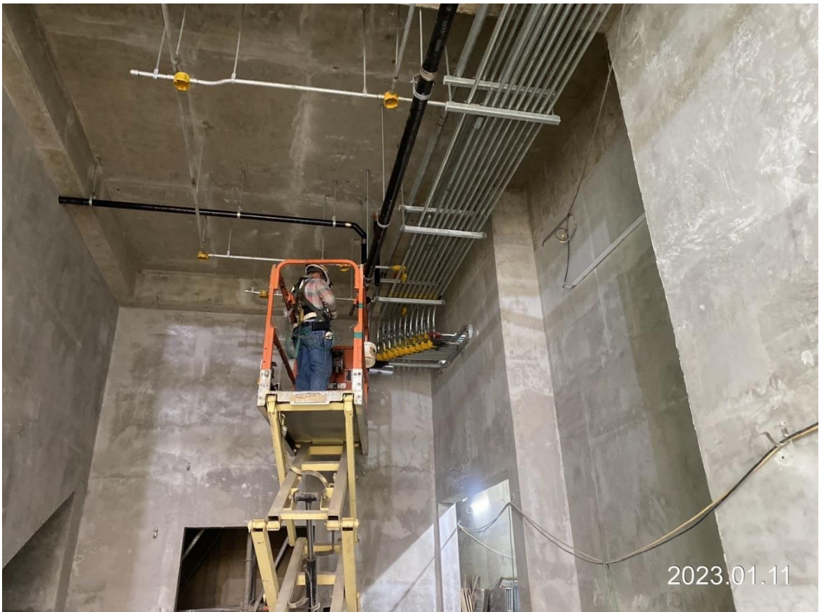
蘆竹中正北路 G13 車站出入口 1 樓排水管施作
