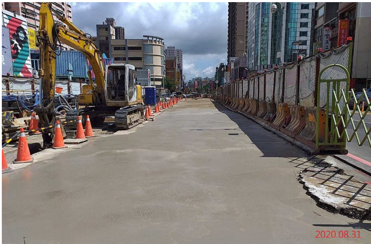
G10 站_北工區連續壁鋪面設置
