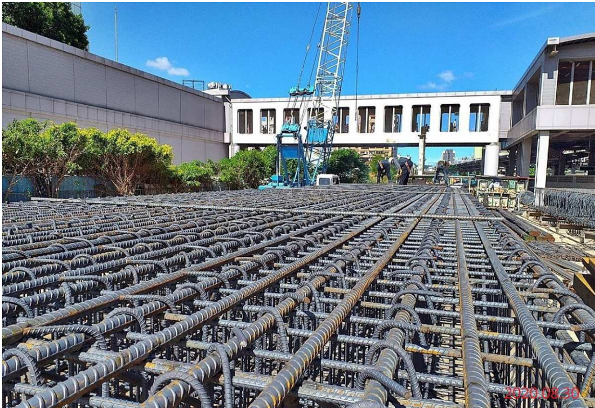
G07 站_連續壁鋼筋籠組立
