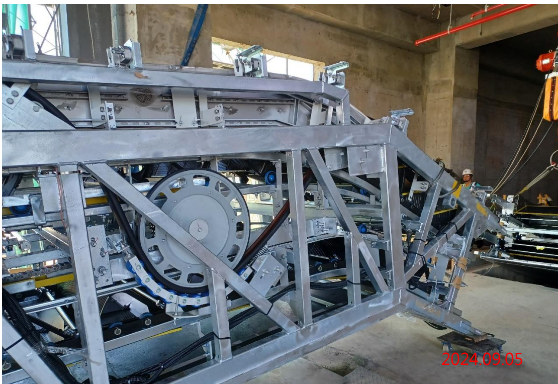
G13a 站-G13-03/04 號電扶梯(出入口二層-出入口三層)吊裝作業
