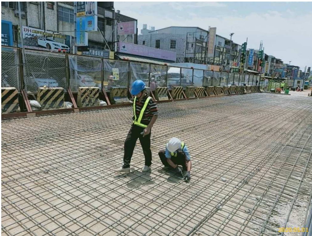
G03 站(巧克力街附近)出入口鋪面鋼筋綁紮
