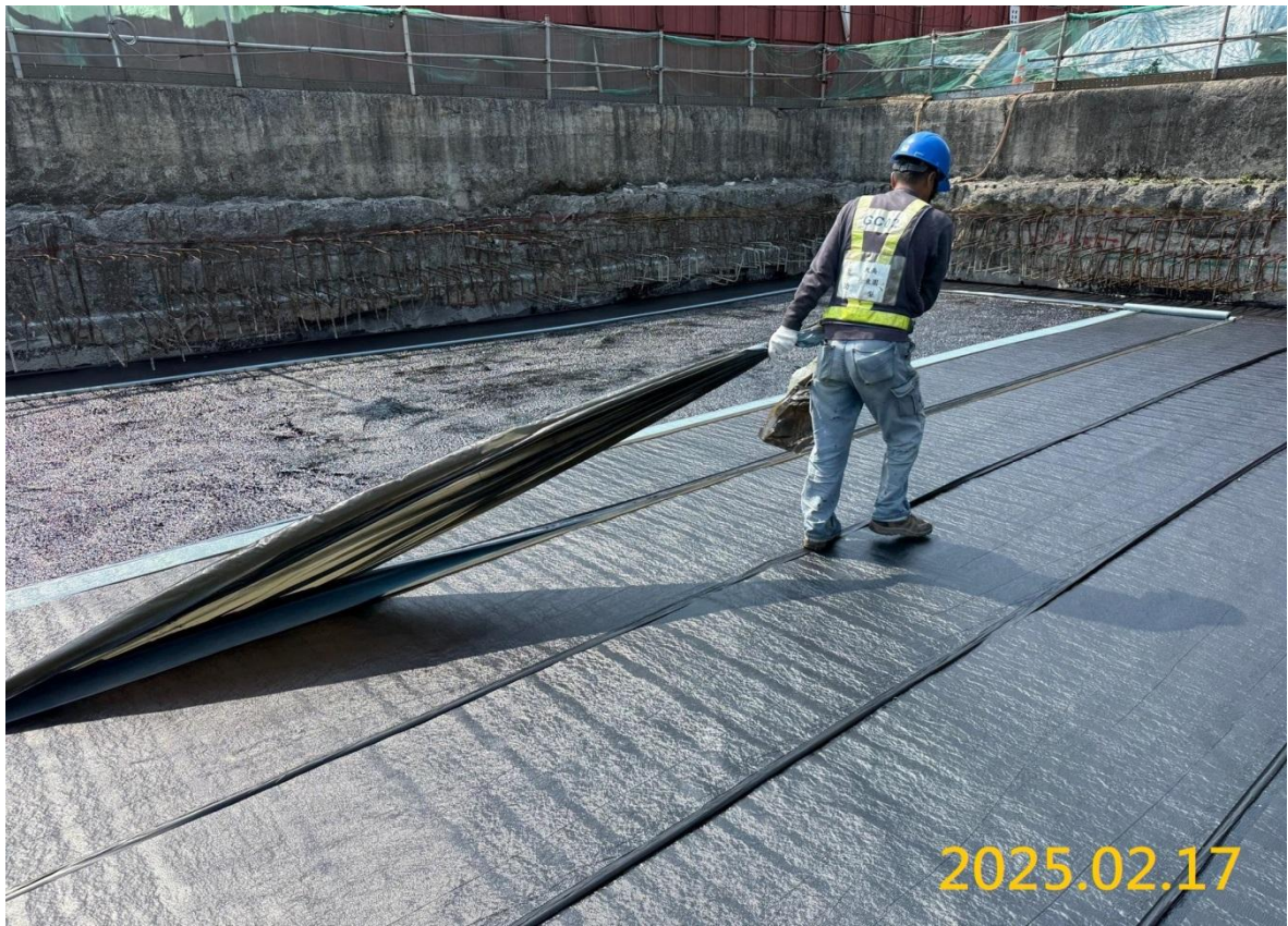
VS6 通風豎井結構頂版防水膜施作
