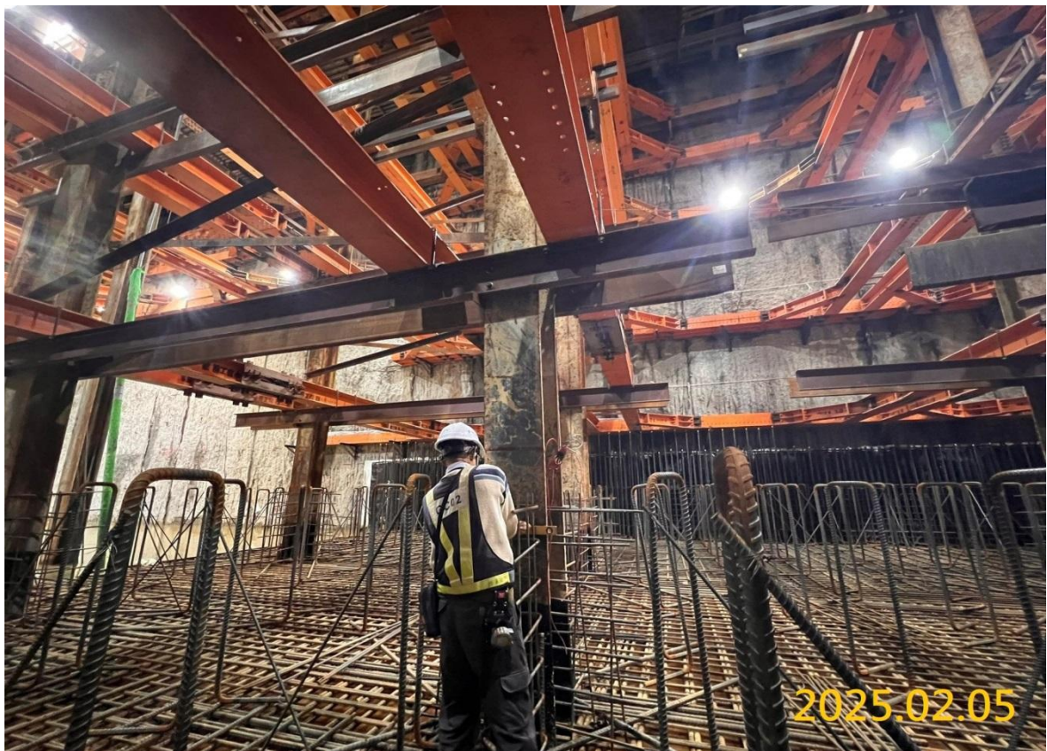
G06 站結構底板施作
