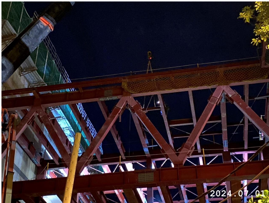
G31 站連通道吊裝 小梁及拉桿安裝
