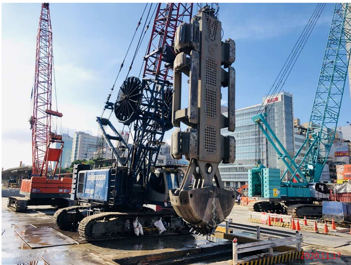
G07 站_連續壁單元抓掘
