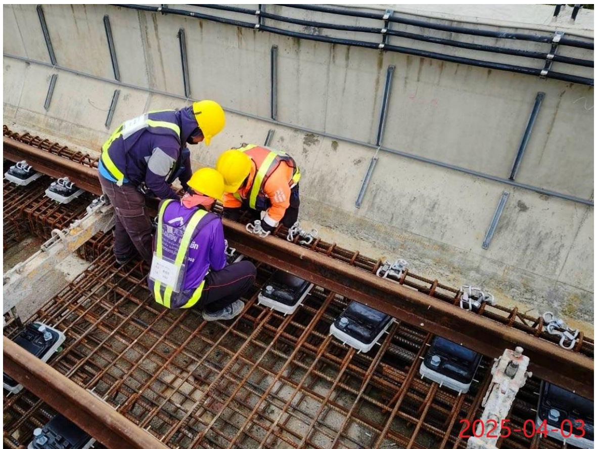
G15-G15a 站間軌道施工
