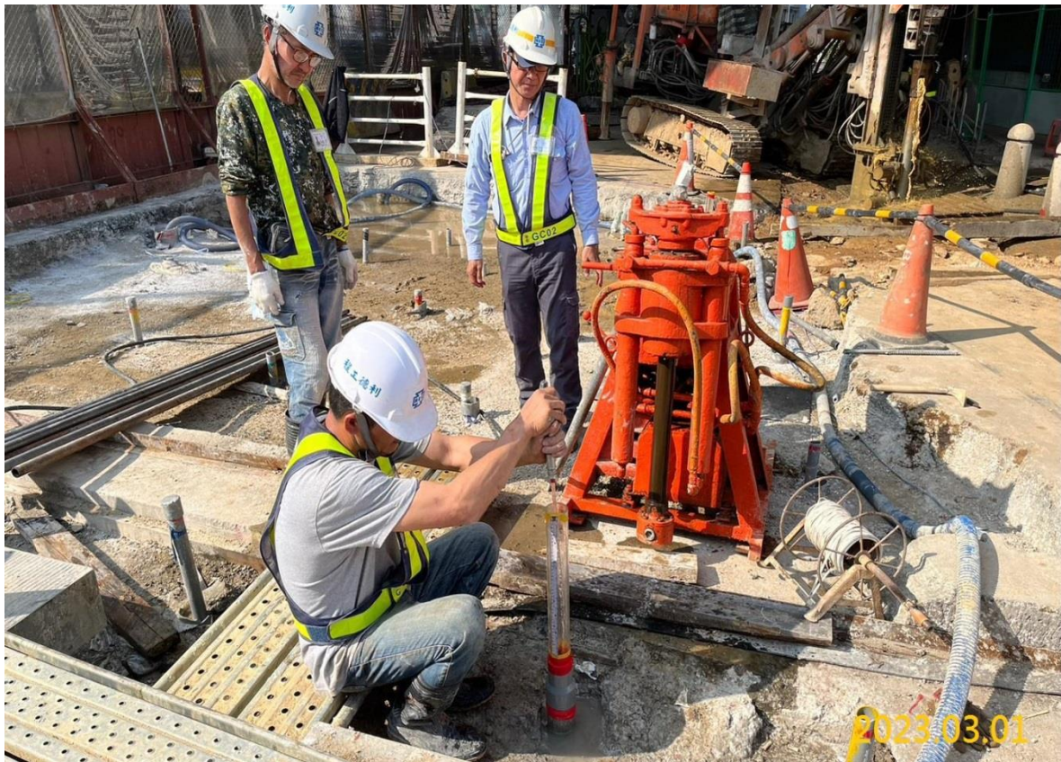
VS5 通風豎井潛盾隧道地盤處理施作
