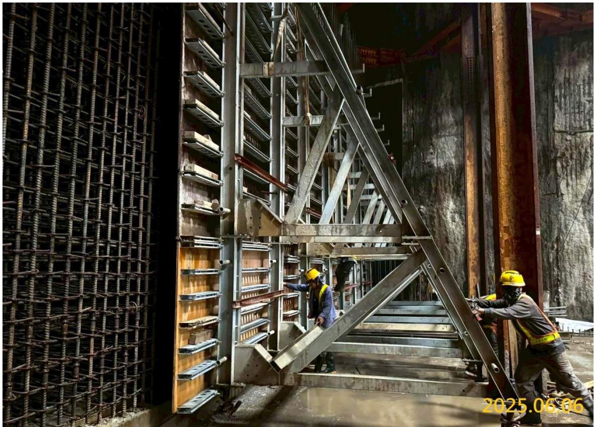
VS5 通風豎井 B2F 結構牆施作
