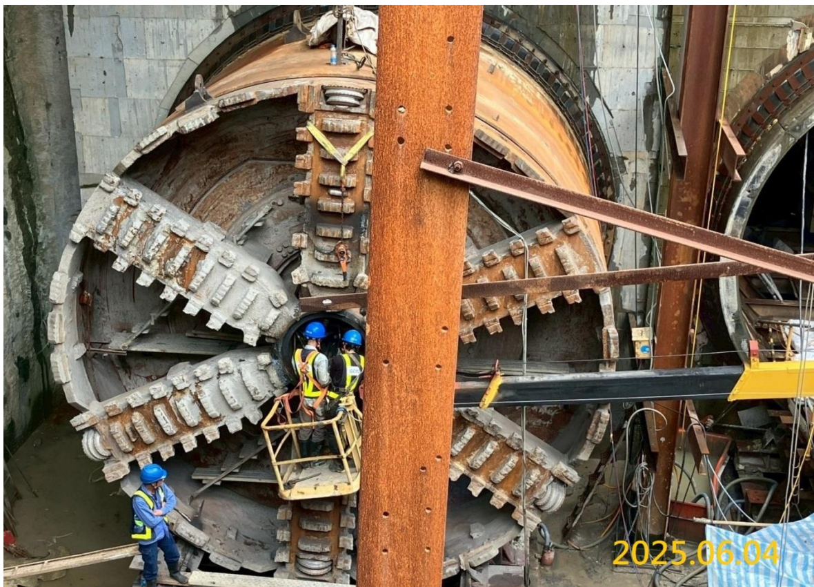
南出土段潛盾隧道到達端潛盾機拆機
