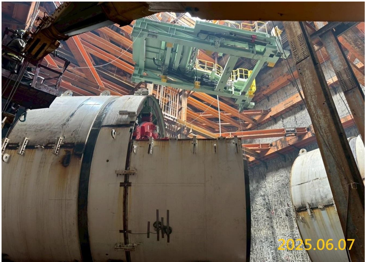
G06 站南井潛盾隧道發進前置作業-潛盾機組裝
