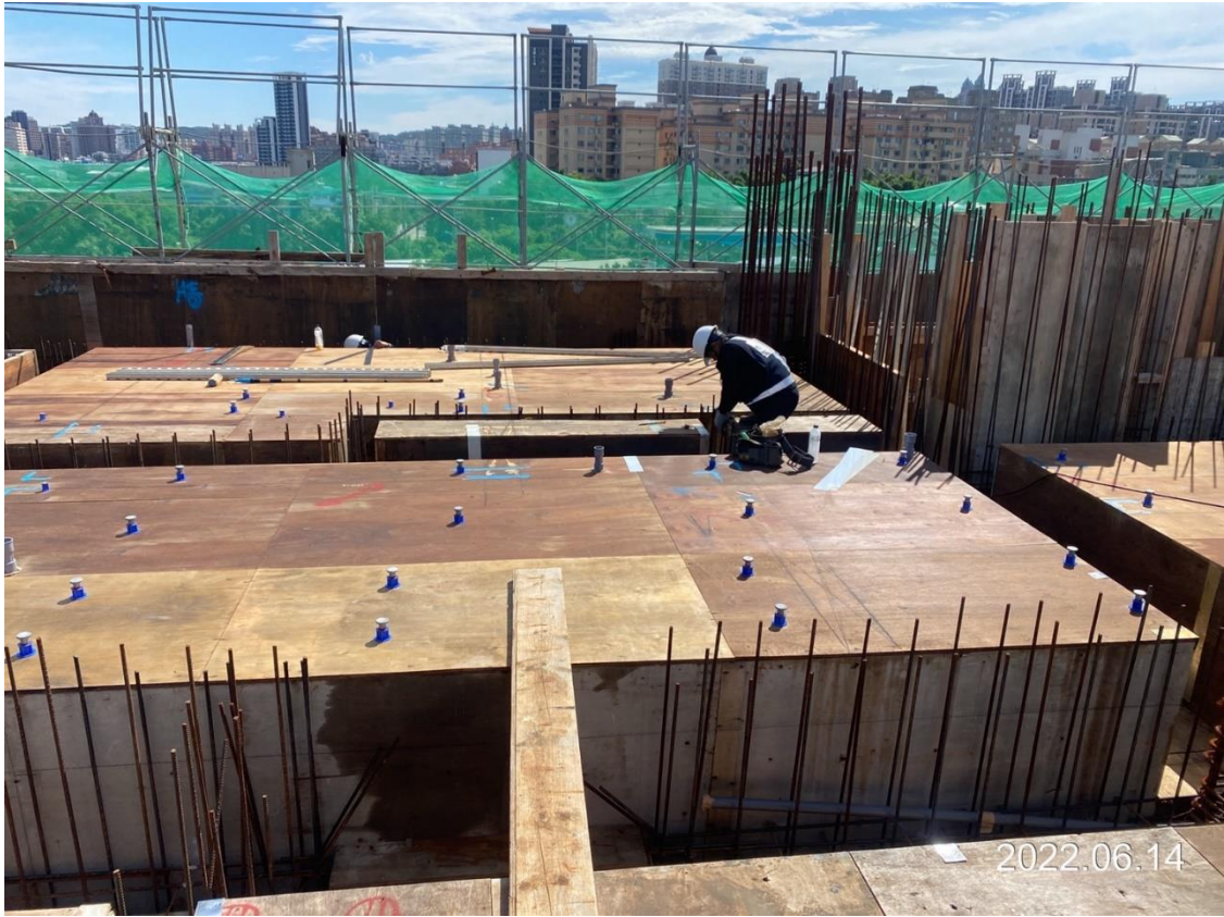
蘆竹中正北路 G13 車站出入口 3 樓版模板組立
