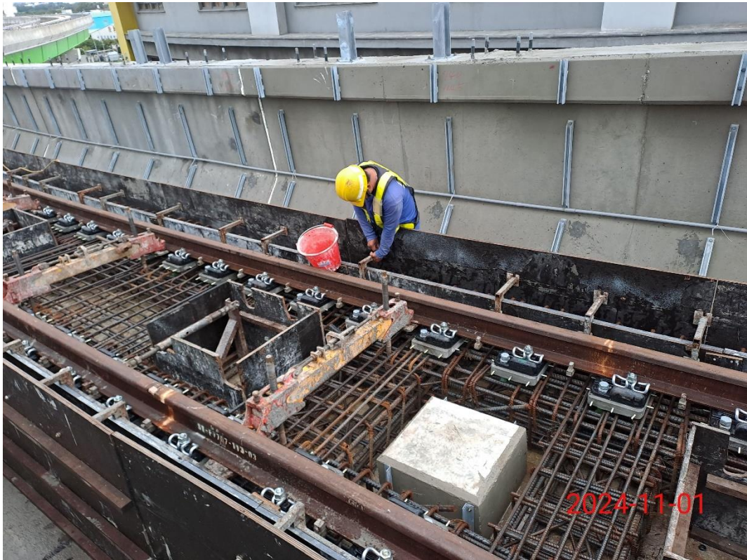
G13a-G14 站間軌道施工
